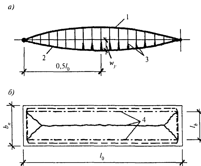
Рис. 13.7. Схема разрушения панели-оболочки КЖС:
