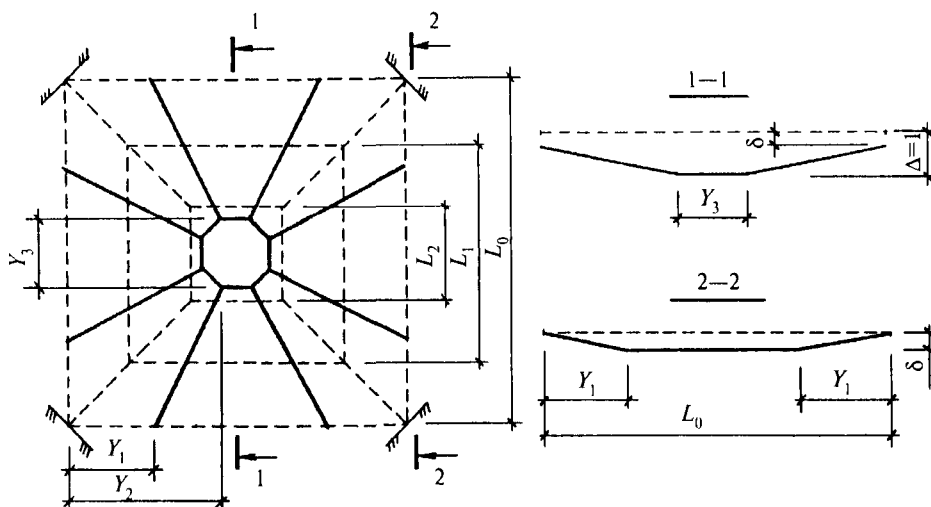
Рис. 15.2. Девятизвенная схема излома
