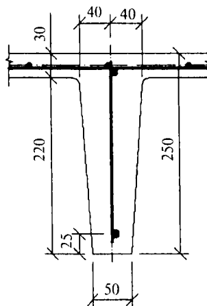
Рис. 8.3. Схема поперечного ребра плиты
