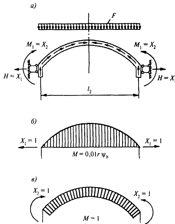
Рис. 7.8. К определению поперечных изгибающих моментов в средней воле длинной цилиндрической оболочки:
