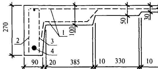
Рис. 14.4. Конструкция панели:
