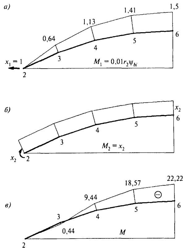
Рис. 5.10. Эпюры моментов в основной системе:
