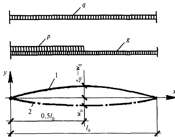
Рис. 13.6. Расчетная схема панели-оболочки КЖС:
