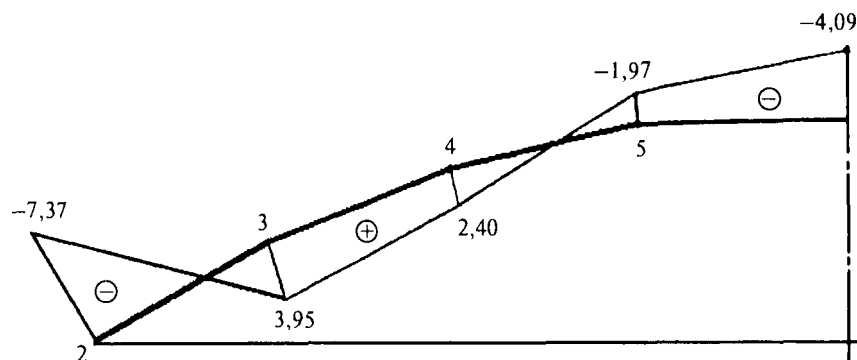
Рис. 5.11. Суммарная эпюра поперечных изгибающих моментов
