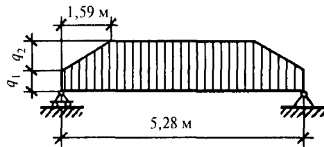
Рис. 14.3. Нагрузка на продольном ребре
