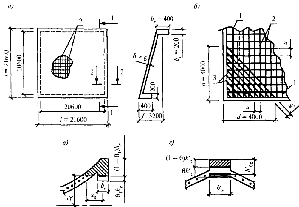
Рис. 11.15. Схема армирования гипара:
