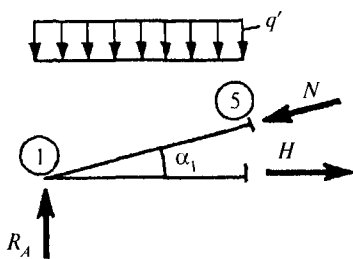
Рис. 11.4. Схема усилий в опорном узле оболочки
