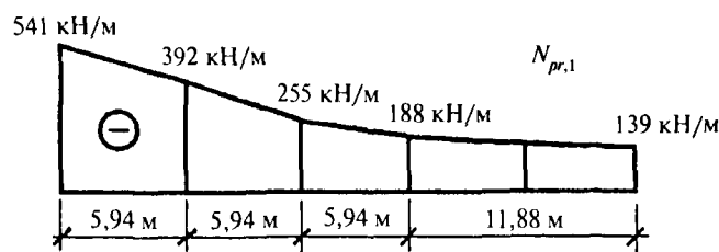
Рис. 10.11. Эпюра N_{pr,1}
