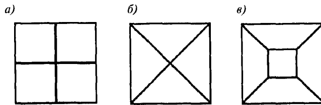
Рис. 15.4. Некоторые частные случаи девятизвеной схемы излома
