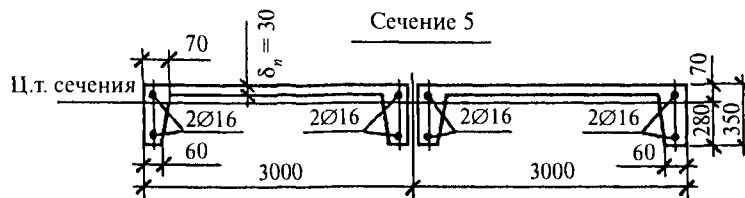
Рис. 11.9. Геометрические размеры шпренгельной системы в сечении 5
