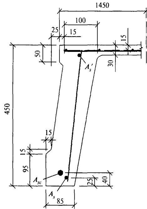
Рис. 8.5. Продольное ребро
