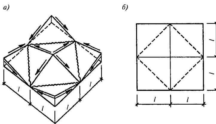
Рис. 11.14. Схема покрытия в форме четырехлепесткового гипара с наклонными коньками: а — общий вид и схема разрушения; б — план покрытия
