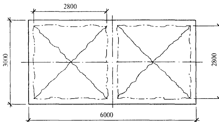
Рис. 10.14. Схема разрушения полки ребристых панелей
