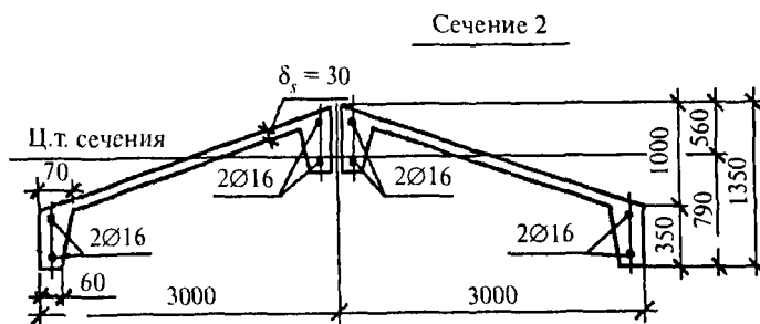
Рис. 11.7. Геометрические размеры шпренгельной системы в сечении 2
