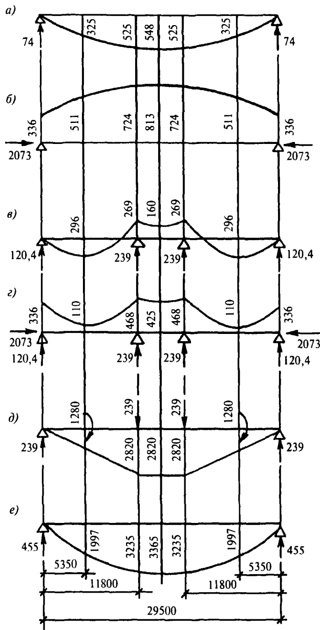
Рис. 7.5. Эпюры изгибающих моментов от нормативных нагрузок, действующих в бортовой балке до замоноличивания (эпюры а–с) и в замоноличенной оболочке (эпюры д, е):
