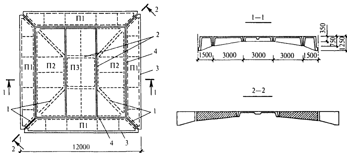
Рис. 15.1. Геометрия сборного рамно-шатрового перекрытия
