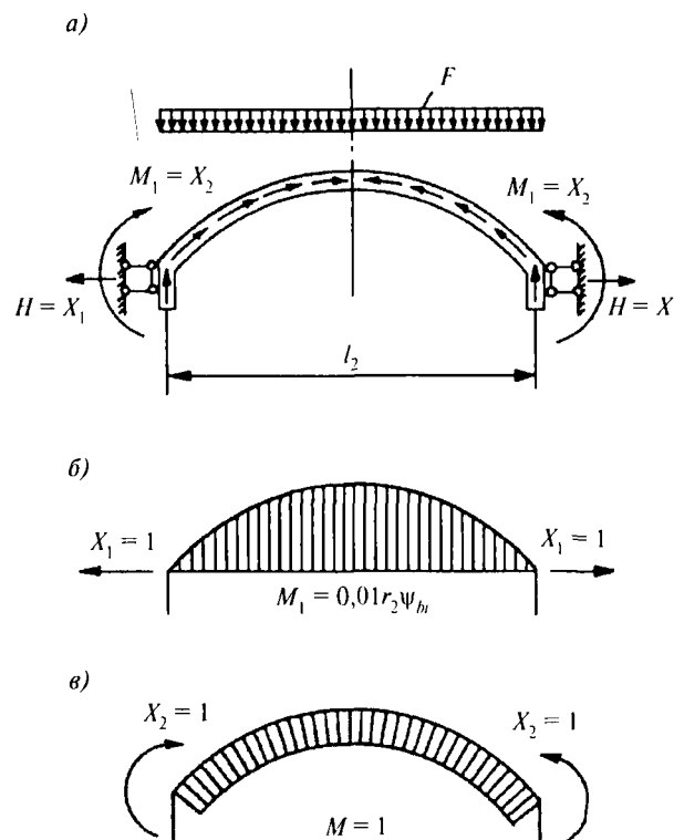
Рис. 5.9. К определению поперечных изгибающих моментов в средней волне свода: а — расчетная схема; б — эпюра моментов от X_1 = 1 ; в — эпюра моментов от X_2 = 1
