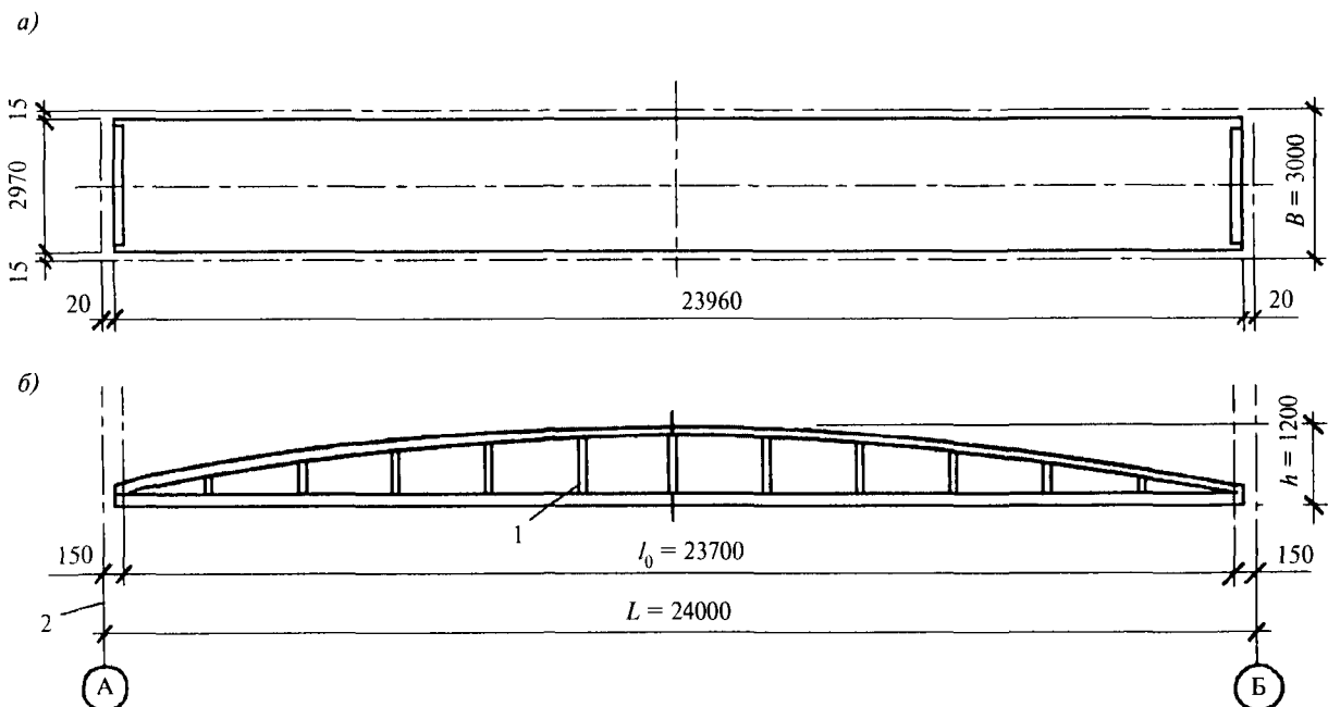
Рис. 13.1. Панель-оболочка КЖС:
