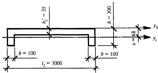
Рис. 10.2. Поперечное сечение цилиндрической плиты
