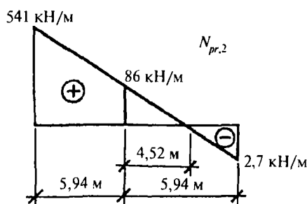
Рис. 10.10. Эпюра N_{pr,2}
