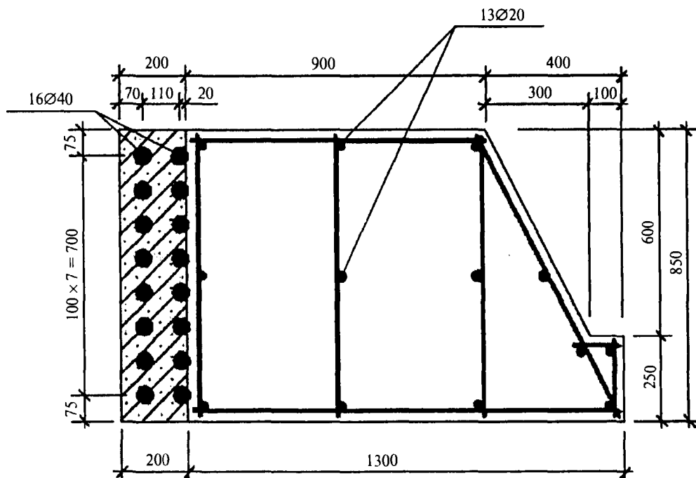
Рис. 9.5. Поперечное сечение и армирование опорного кольца купола
