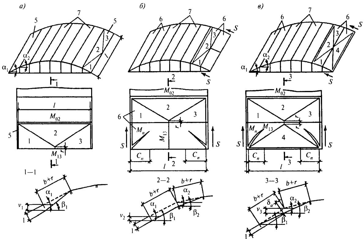
Рис. 8.2. Схемы излома складчатого покрытия:
