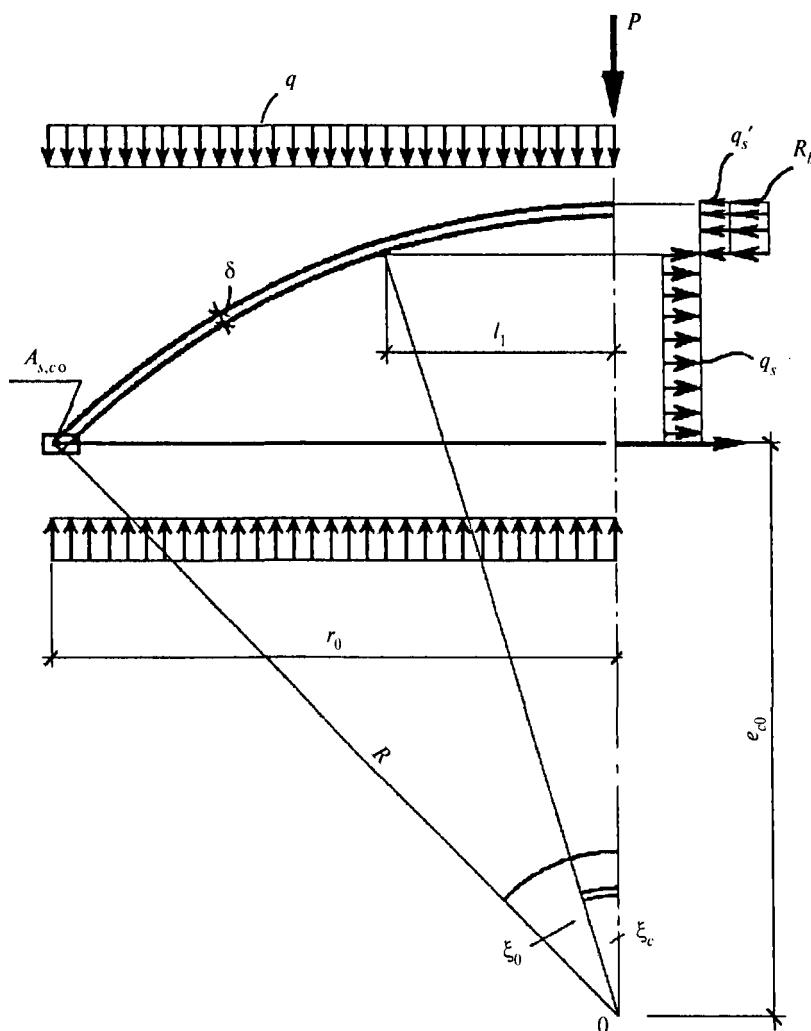
Рис. 9.8. К расчету купола по «балочной» схеме
