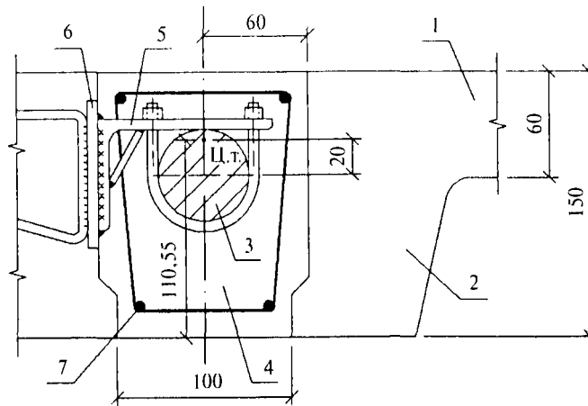
Рис. 12.2. Схема расположения ванты в продольном шве между плитами:
