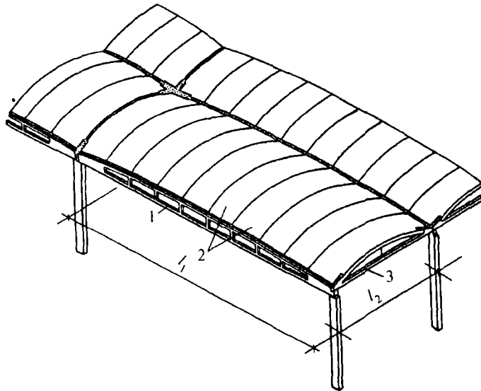
Рис. 7.1. Длинная цилиндрическая оболочка:
