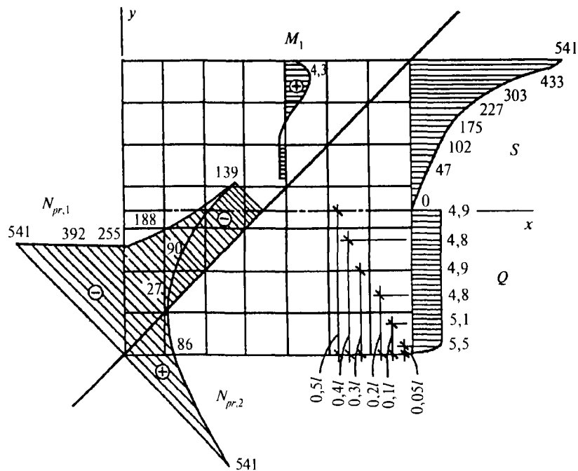
Рис. 10.5. Эпюры усний M , S , Q , N_{pr}
