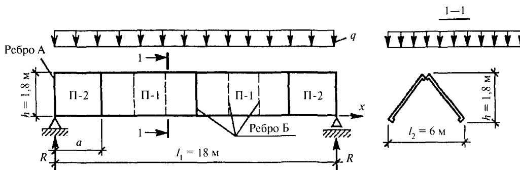
Рис. 6.1. Конструктивная схема складки из ребристых плит
