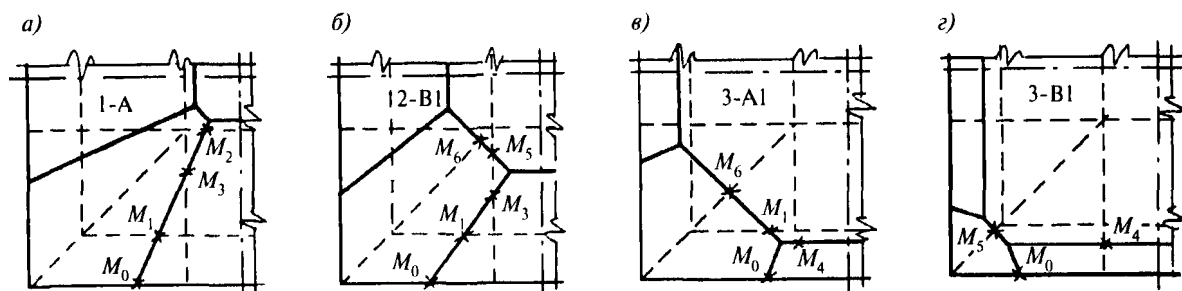
Рис. 15.3. Некоторые расчетные случаи вычисления работы внутренних сил
