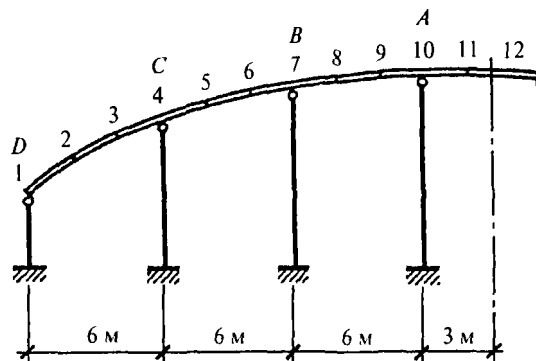
Рис. 10.16. Схема разбивки контура на участки
