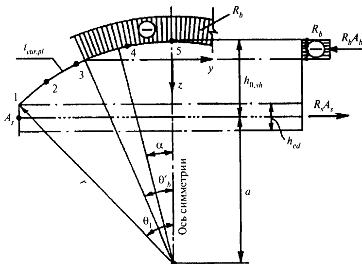
Рис. 7.3. Схема усилий и эпюра напряжений в сечении, нормальном к продольной оси изгибаемой цилиндрической оболочки, при расчете по прочности
