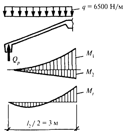
Рис. 6.5. Эпюра расчетного изгибающего момента M_t
