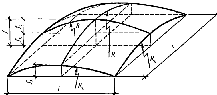
Рис. 10.1. Схема оболочки
