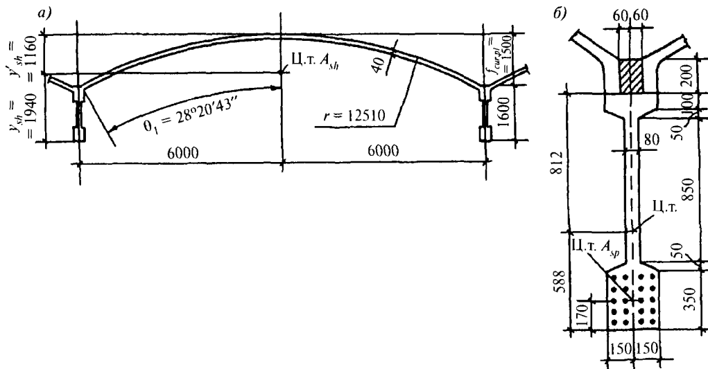
Рис. 7.2. Геометрические размеры цилиндрической оболочки:
