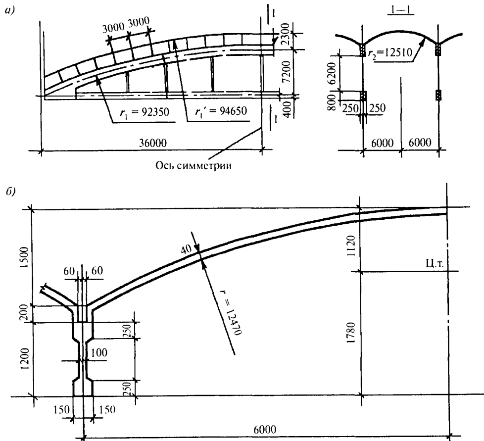
Рис. 5.1. Схема многоволнового свода пролетом 72 м:
