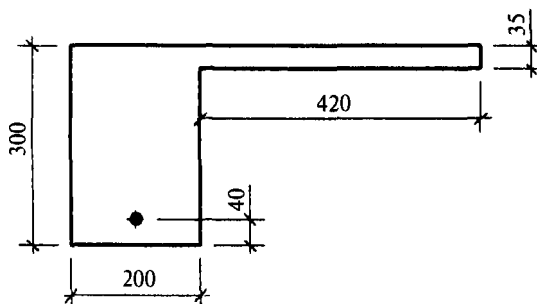
Рис. 10.13. Поперечное сечение плиты (на два ребра)
