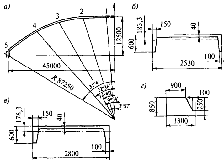
Рис. 9.1. Расчетное сечение купола:
