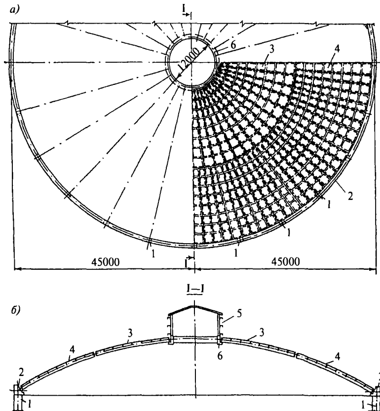
Рис. 9.2. Конструкция купола:
