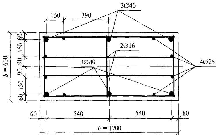
Рис. 12.3. Поперечное сечение и армирование опорного кольца
