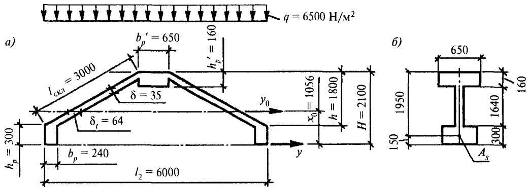
Рис. 6.3. Приведенные поперечные сечения складки: а — в виде двух плит; б — в виде двутавра
