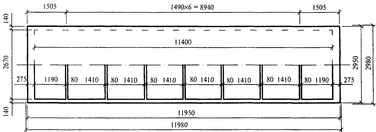
Рис. 8.4. План плиты 3×12 м
