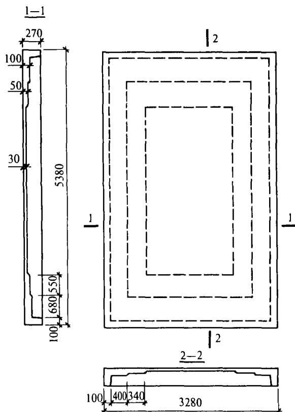
Рис. 14.1. Геометрия панели
