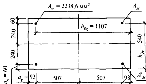
Рис. 12.4. Приведение армирования опорного кольца к симметричному в виде четырех угловых стержней
