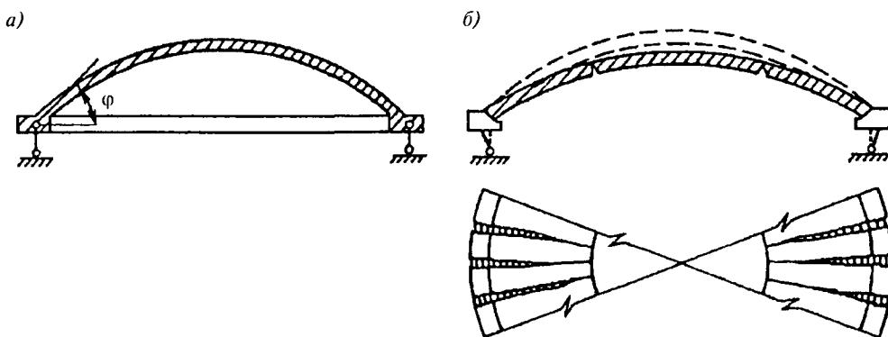
Рис. 9.7. К расчету купола по предельному равновесию: а — поперечное сечение; б — схема разрушения
