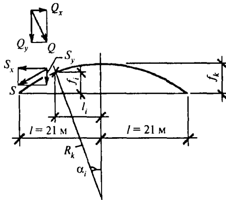
Рис. 10.17. Схема усилий S и Q , действующих на контуре
