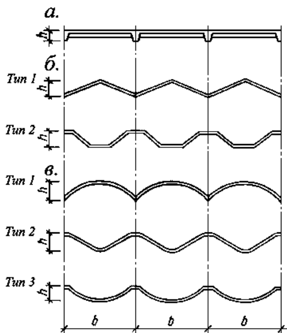
a — цилиндрические своды; б — складчатые своды (типы 1 и 2); в — волнистые своды (типы 1, 2, 3)
