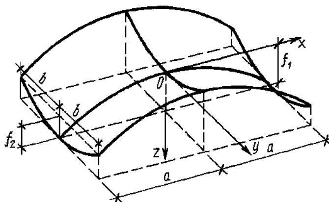
Рисунок 12.1. Гиперболический параболоид
