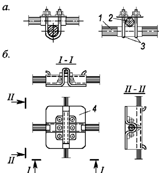
1 — несущая ванта; 2 — напрягающая ванта; 3 — хомут; 4 — косынка.
