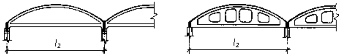
Рисунок 9.12. Диафрагмы цилиндрических оболочек
