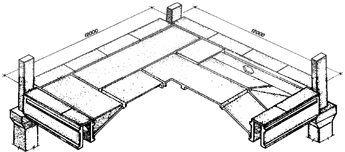
Рисунок 16.6. Ячейка сборного шатрового перекрытия под тяжелые нагрузки
