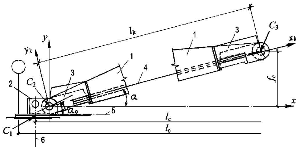
1 – панель оболочки КЖС; 2 – упор затяжки; 3 – закладная деталь с отверстием для шарнира; 4 – рабочей арматуры диафрагм; 5 – ось затяжки; 6 – ось опорной конструкции.
