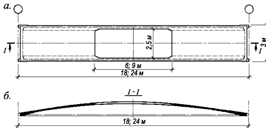
a — план; б — продольный разрез по оси панели
