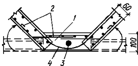
1 — бетон замоноличивания; 2 — отгибаемые и свариваемые выпуски; 3 — предварительно напряженная арматура, натягиваемая на упоры формы; 4 — дополнительные сетки.
