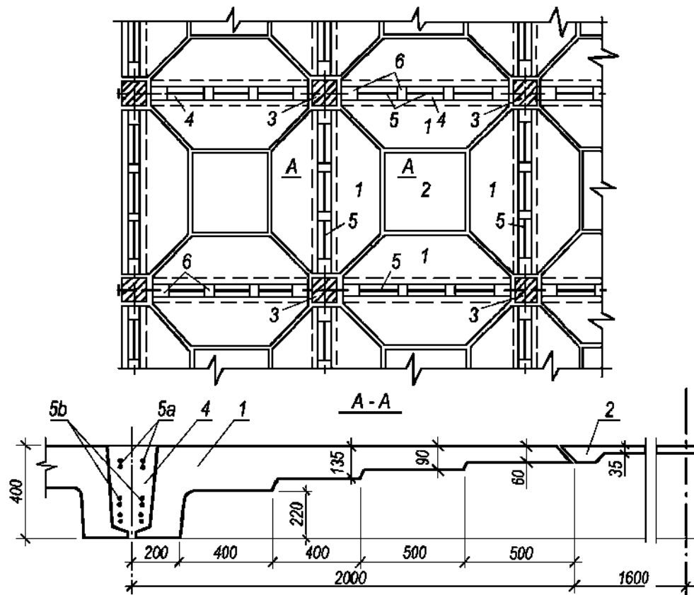
Рисунок 15.6. Схема неразрезного сборного перекрытия с предварительно напряженной арматурой, уложенной в швы между панелями
