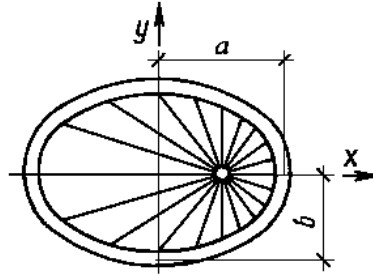
Рисунок 13.12. Радиально-вантовая система с узлом в фокусе эллипса
