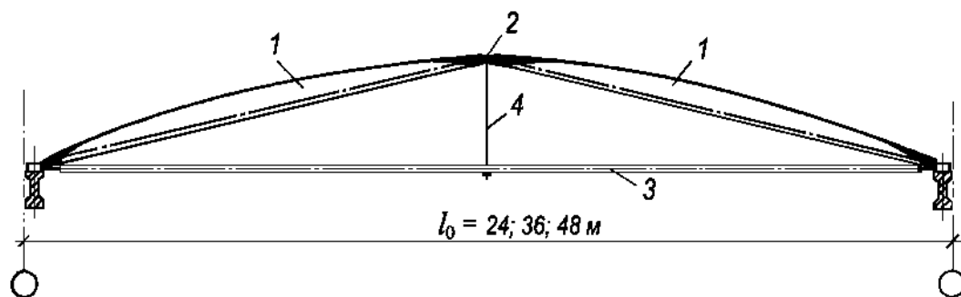
Рисунок 14.10. Конструктивная схема сегментного свода для покрытий, опирающегося на продольные балки каркаса здания
