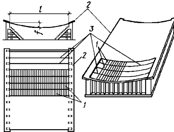
Рисунок 13.1. Висячая оболочка с параллельной системой вант
