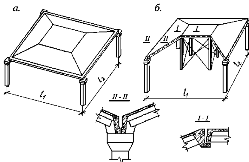
a — из шатровых элементов размером на ячейку здания; б — из унифицированных элементов с использованием сборочного кондуктора.
