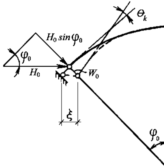
Рисунок 10.2. Расчетная схема узла сопряжения опорного кольца и оболочки купола
