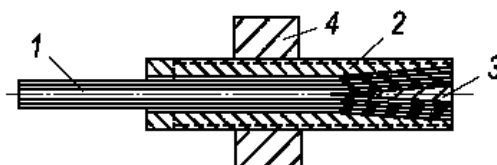
Рисунок 13.10. Гильзотуповой анкер для вант из высокопрочной проволоки и стальных канатов
