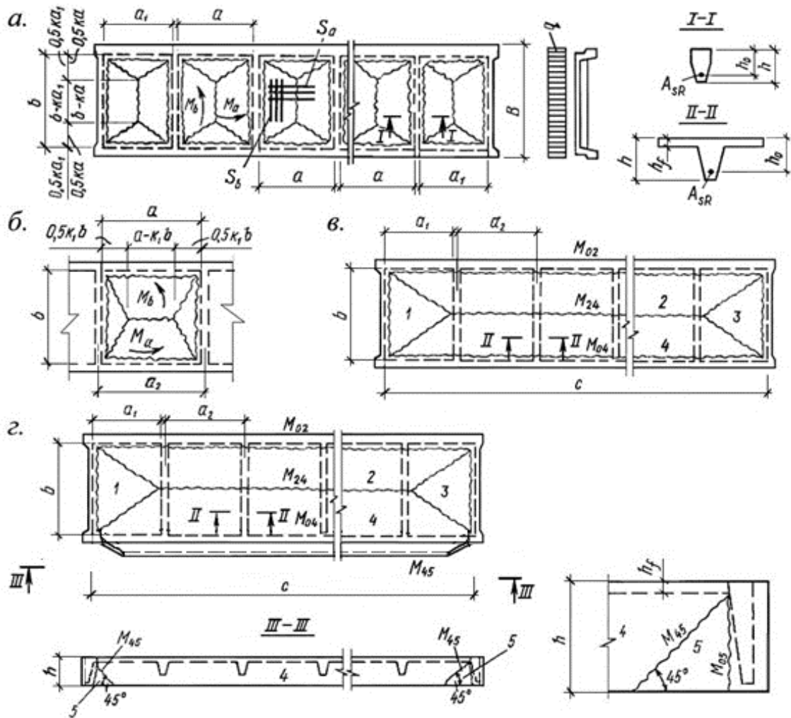
а, б, в — схемы разрушения для всех плит; г — то же, для крайних плит; 1...5 — диски в схемах разрушения
