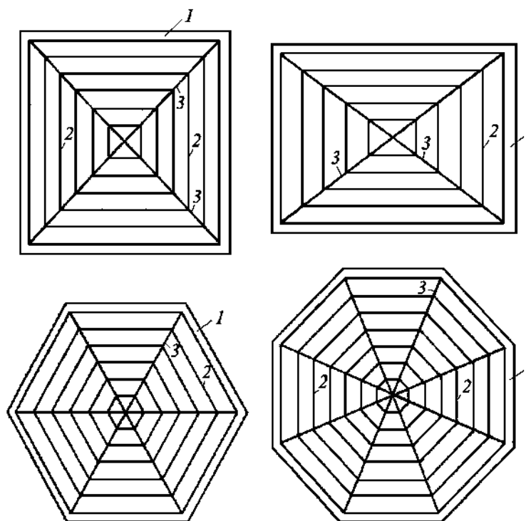
Рисунок 13.4. Висячие оболочки с перекрестной системой вант
