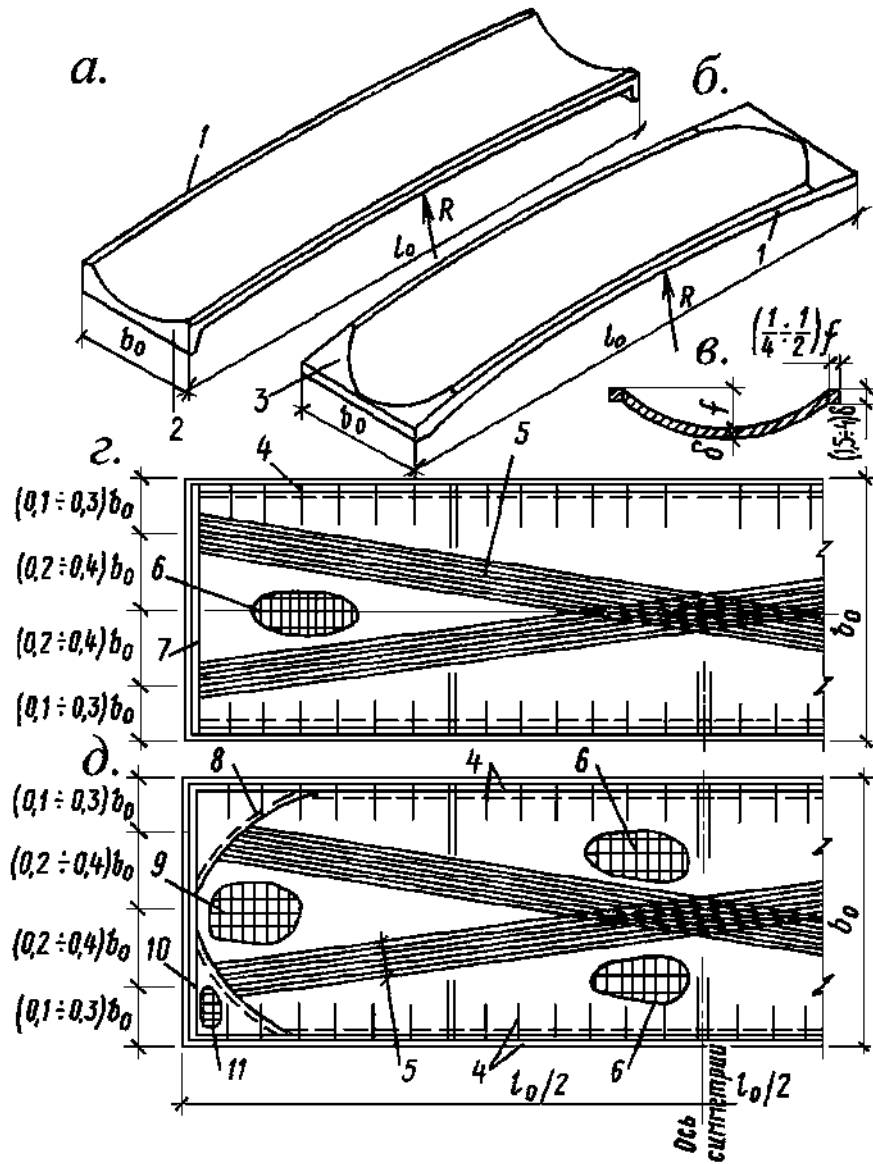
a — с вертикальными торцевыми диафрагмами; б — то же, с наклонными; в — поперечное сечение панели; г — план армирования панели с вертикальными торцевыми диафрагмами; д — то же, с наклонными; 1 — продольный борт; 2 — диафрагма вертикальная; 3 — то же, наклонная; 4 — каркас продольного борта; 5 — предварительно напряженная холоднодеформированная арматура периодического профиля (арматурные канаты); 6 — сварная сетка оболочки; 7 — арматура торцевой диафрагмы.
