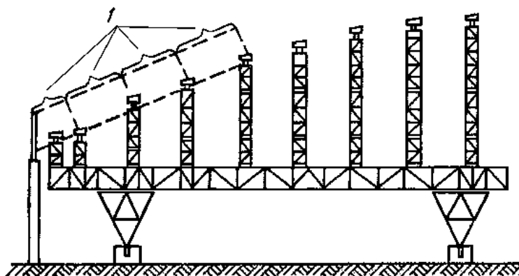
1 — укрупненные монтажные блоки.
