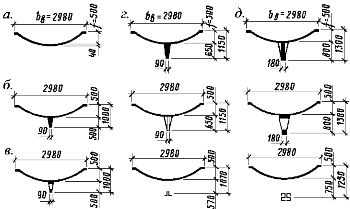
a — пролетом 12 м; б, в — то же, 18 м (со сплошным килем и с отверстиями в нем); з — то же, 21 м (со сплошным и облегченным килем и с затяжкой); д — то же, 24 м (с облегченным килем, с отверстиями в нем и с затяжкой).
