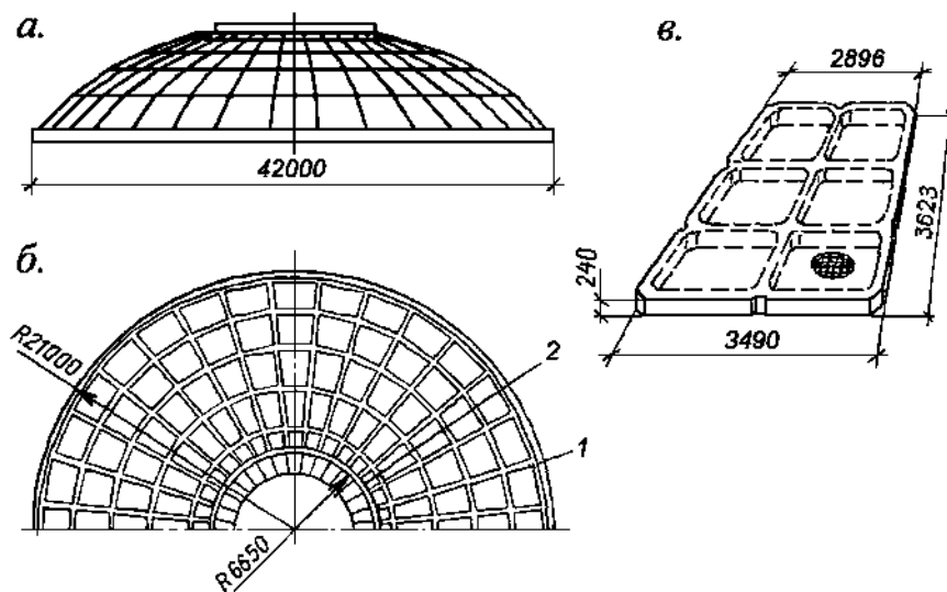
Рисунок 10.11. Сборный купол из плоских ребристых плит
