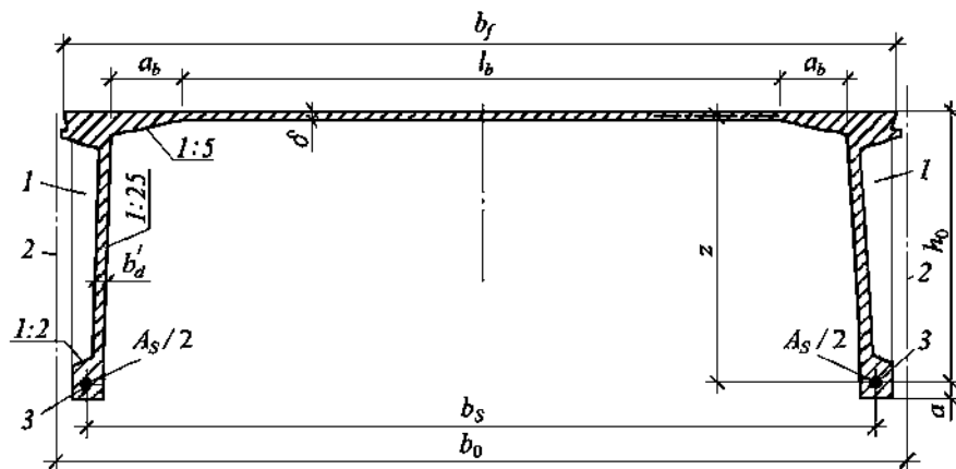
Рисунок 14.2. Поперечное сечение панели-оболочки КЖС
