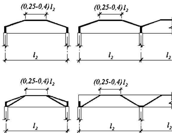
Рисунок 9.2. Типы складчатых оболочек
