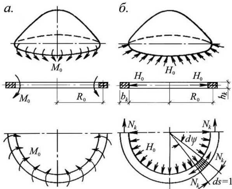
Рисунок 10.4. Момент и распор при взаимодействии оболочки и опорного кольца купола
