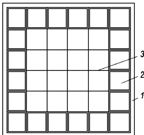
1 — опорный контур; 2 — плита; 3 — ванты
