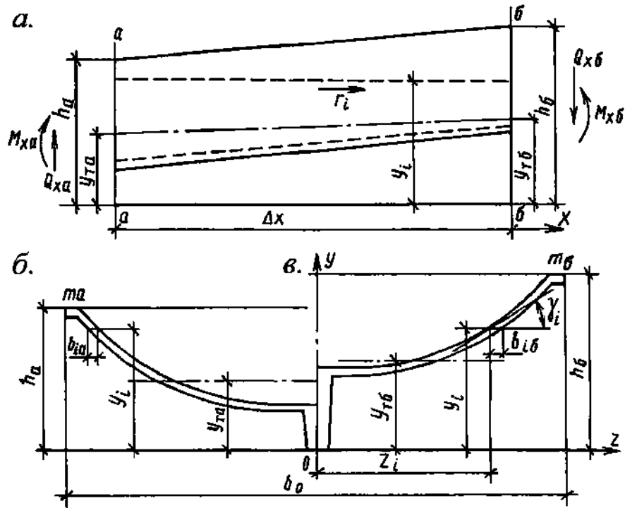
a — элемент длиной \Delta x ; б — половина поперечного сечения a—a ; в — то же, поперечного сечения б—б .
