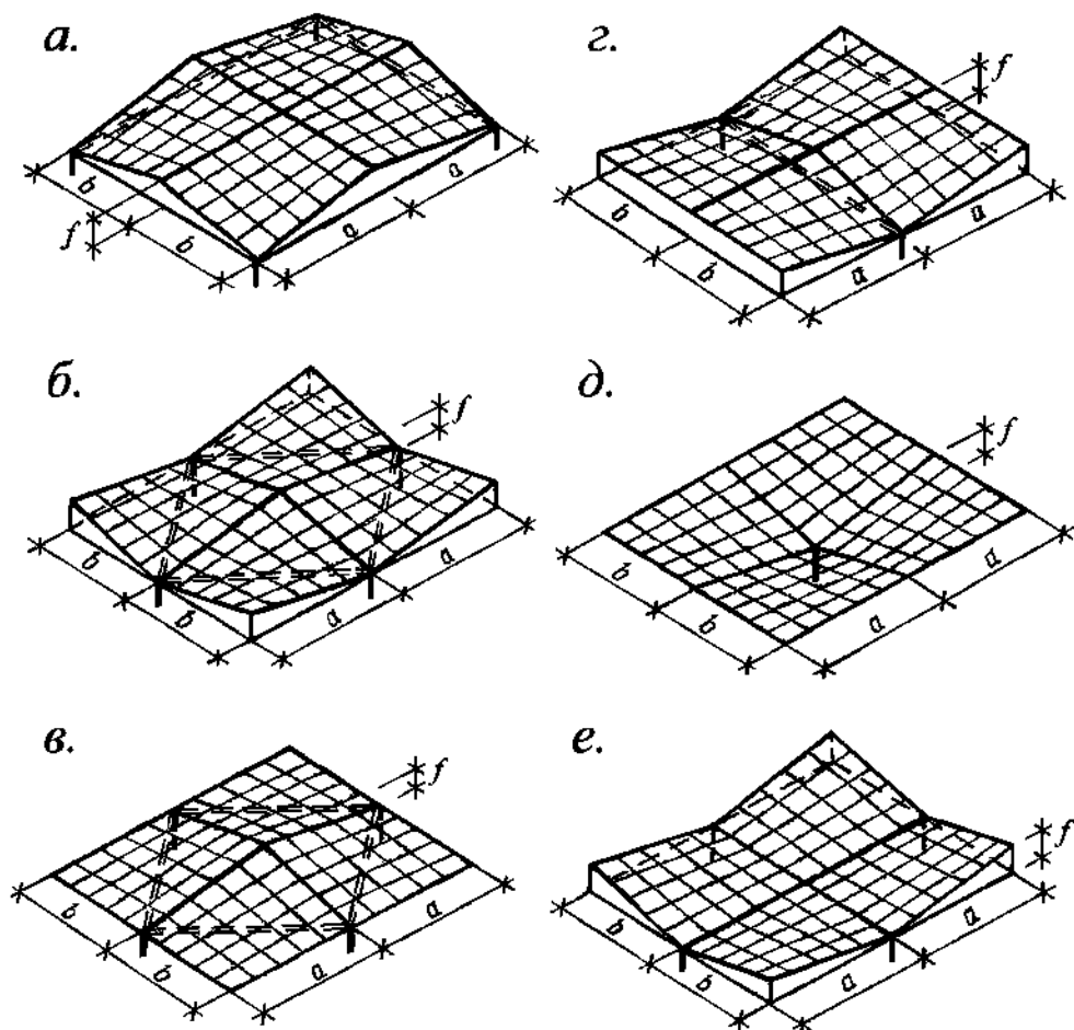
Рисунок 12.3. Четырехлепестковые гипары
