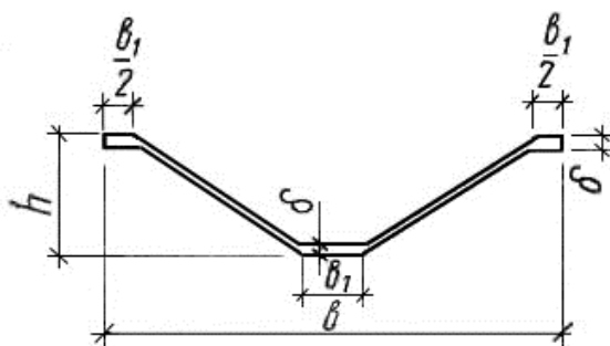
Рисунок 7.13. Трапецевидное поперечное сечение элемента свода
