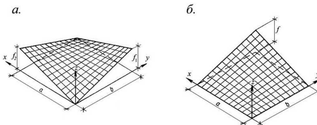
Рисунок 12.2. Однолепестковые гипары
