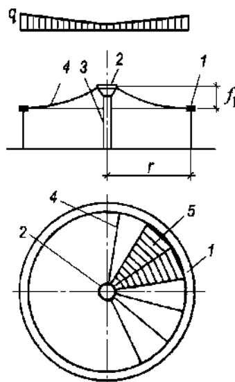
Рисунок. 13.3. Шатровая висячая оболочка
