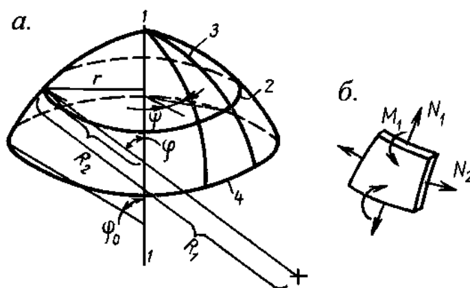
a — геометрия; б — схема усилий; 1 — ось вращения; 2 — параллель; 3 — меридиан; 4 — краевой параллельный круг.
