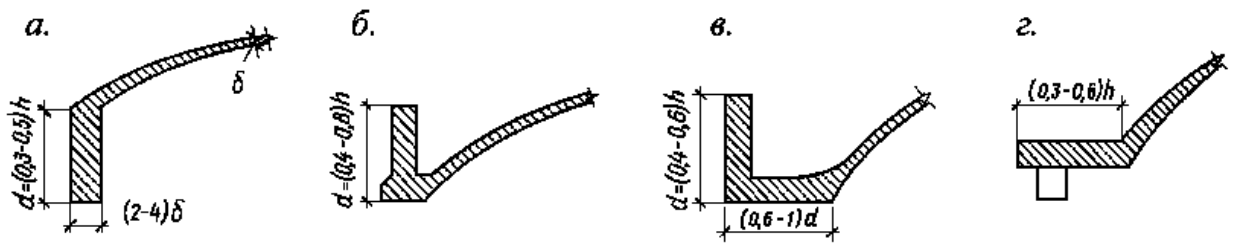
Рисунок 9.11. Бортовые элементы
