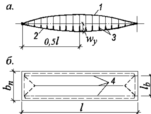
a — вид на диафрагму; b — план; 1 — оболочка; 2 — рабочая арматура диафрагм; 3 — трещины в диафрагме; 4 — пластические шарниры в оболочке
