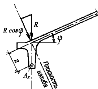
Рисунок 16.5. Расчетная плоскость изгиба крайних элементов шатровых складок
