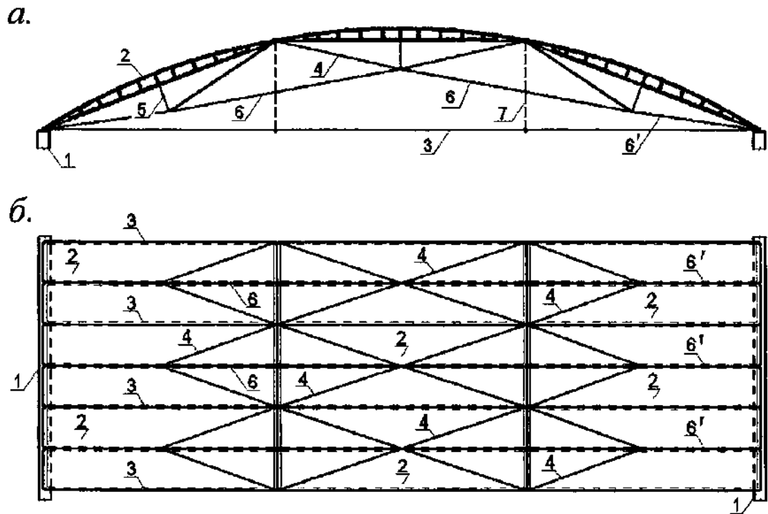
a – вид сбоку; б – план свода, состоящего по длине из 6 панелей-оболочек КЖС; 1 – опорная конструкция; 2 – панели-оболочки КЖС; 3 – затяжки; 4 – наклонные связи, образующие в плане ромбическую систему связей; 5 – стойки, снабженные натягающим устройством; 6 – дополнительные стержни, соединяющие нижние углы треугольной решетки; 6' – опорная связь треугольной решетки.
