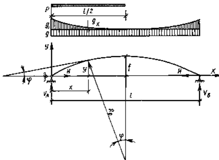
Рисунок 7.4. Расчетная схема свода
