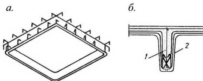
a — тонкостенный коробчатый железобетонный или армоцементный элемент; б — деталь поперечного сечения конструкции; 1 — монолитный бетон; 2 — выпуски арматуры из несущей опалубки.
