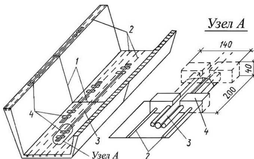
1 — линия стыка; 2 — предварительно напряженная арматура элемента; 3 — предварительно напряженные вставки; 4 — анкерные колодки.
