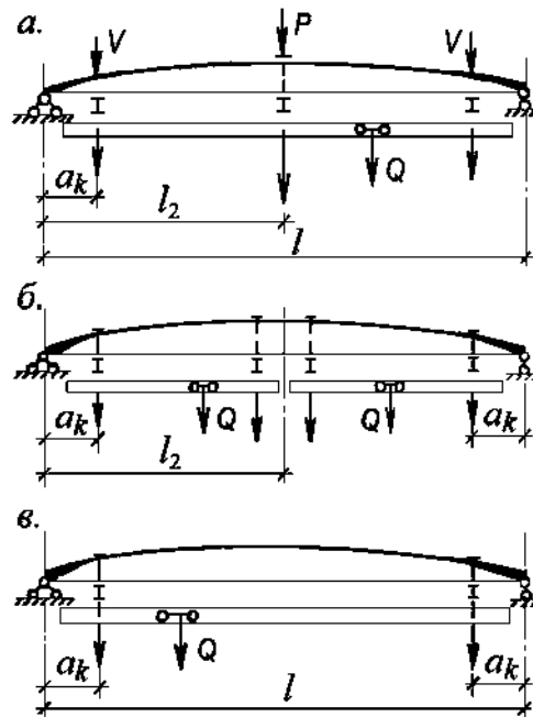
Рисунок 14.8. Типовые схемы нагружения (а, б, в) покрытия из панелей-оболочек КЖС подвесными кранами
