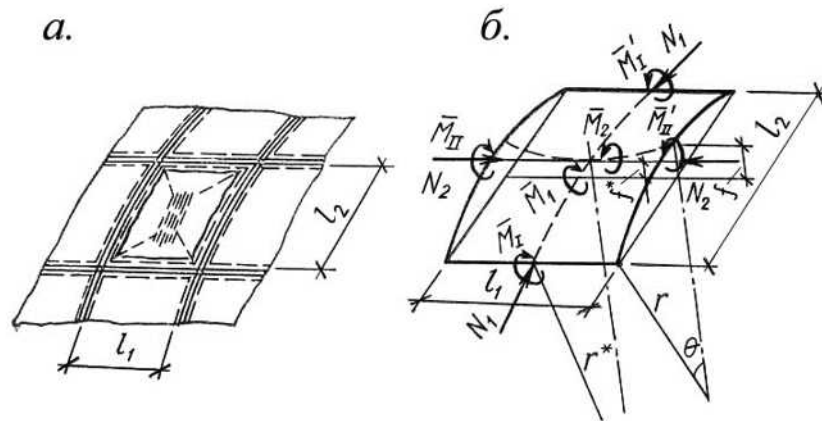
a — схема разрушения плиты между ребрами; б — взаимодействие усилий на контуре зоны разрушения
