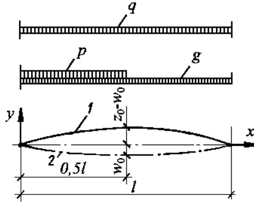
Рисунок 14.6. Расчетная схема панели-оболочки КЖС
