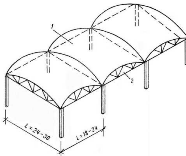
1 — монолитная плита-оболочка; 2 — металлическая или сборная железобетонная ферма-диафрагма
