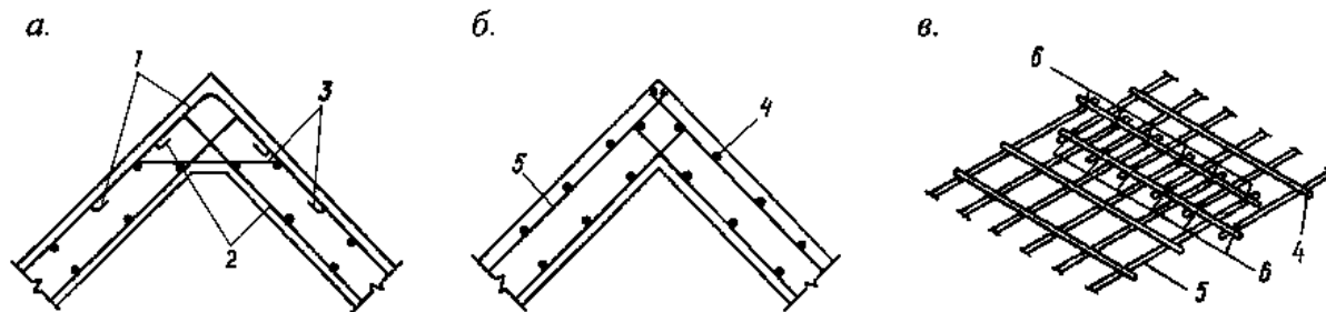
a — отдельными стержнями; б — сварными сетками; в — положение сеток при сварке; 1 — верхние стержни; 2 — то же, нижние; 3 — армирование в вутах; 4 — поперечные стержни пересекающихся сеток; 5 — то же, продольные; 6 — места точечной сварки.
