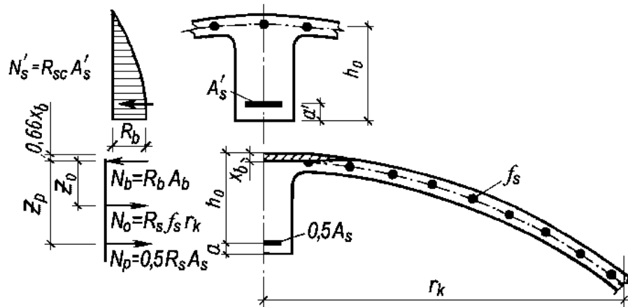
Рисунок 11.19. Схема взаимодействия усилий в радиальном сечении оболочек.
