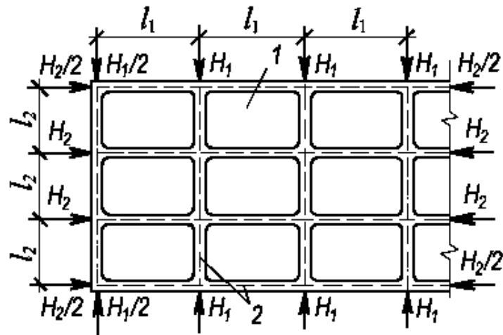
Рисунок 15.6. Схема неразрезного сборного перекрытия с предварительно напряженной арматурой, уложенной в швы между панелями
