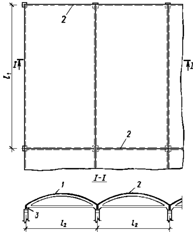
Рисунок 9.1. Цилиндрические оболочки
