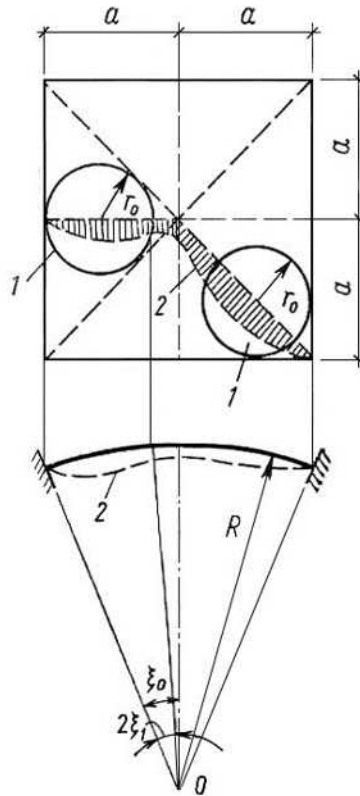
Рисунок 11.13. Схема разрушения оболочки с образованием локальной вмятины
