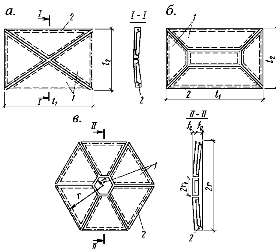
а — на прямоугольном плане из треугольных элементов; б — на прямоугольном плане из прямоугольного и трапециевидных элементов; в — на полигональном контуре; 1 — сборные панели; 2 — арматурный пояс.
