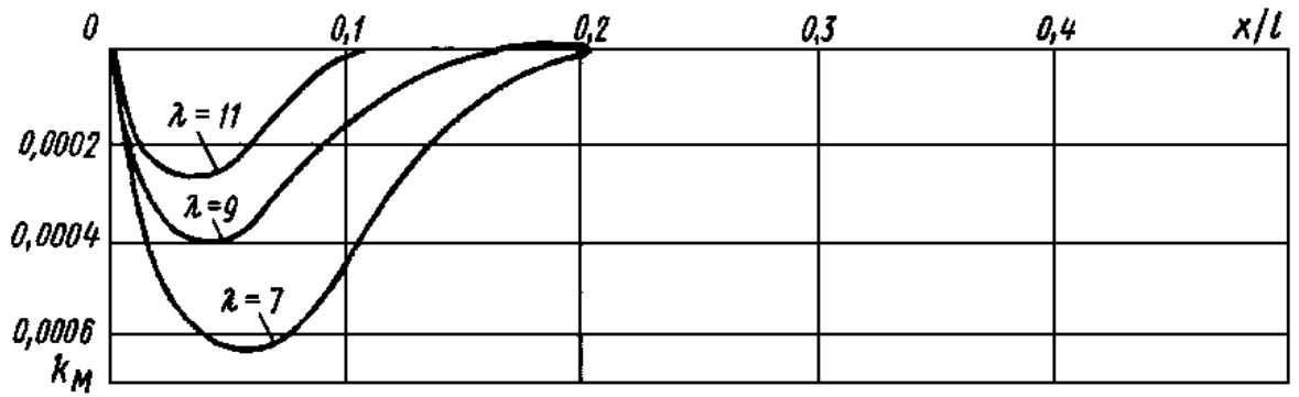
Рисунок 11.7. Графики коэффициентов k_M
