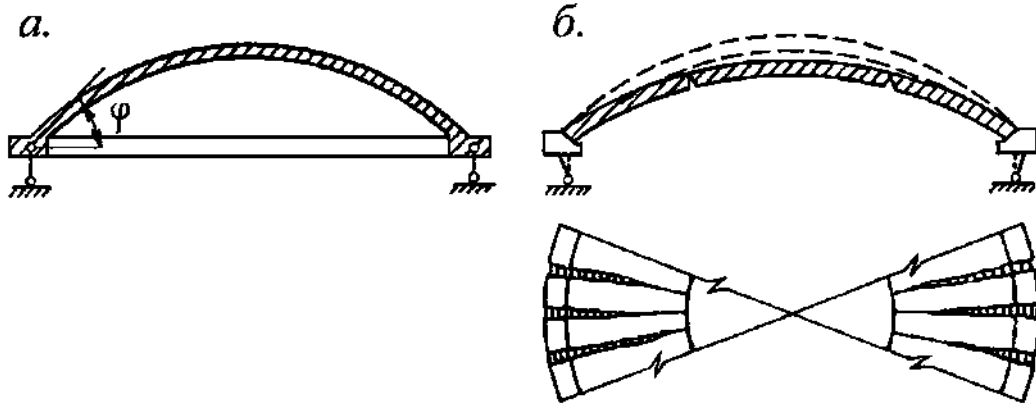
a — поперечное сечение; б — схема разрушения.
