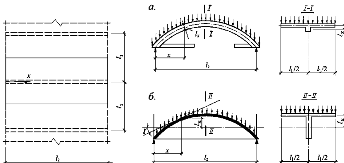
a — арочной; б — балочной
