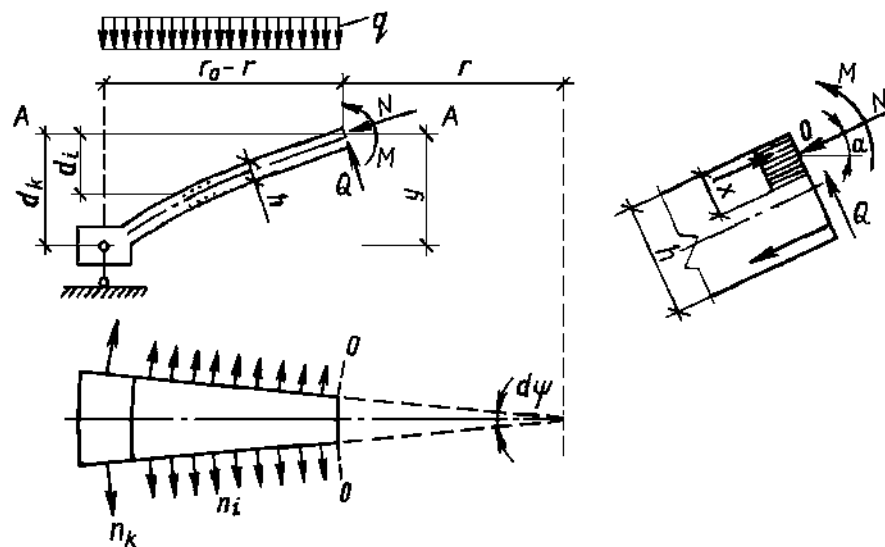
Рисунок 10.6. Схема взаимодействия усилий в куполе в предельном состоянии
