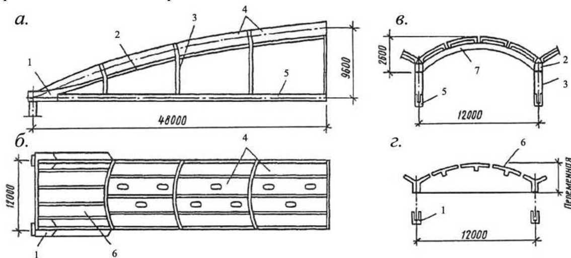
а – продольный разрез по своду; б – план раскладки плит; в – поперечный разрез по средней зоне; 2 – то же по опорной зоне; 1 – опорный блок; 2 – бортовые элементы; 3 – стальная подвеска; 4 – средняя плита с отверстиями; 5 – блок затяжки; 6 – плита опорной зоны; 7 – балка диафрагмы.
