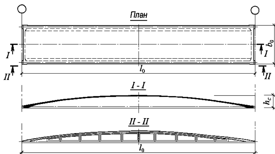
Рисунок 14.1. Панель-оболочка КЖС
