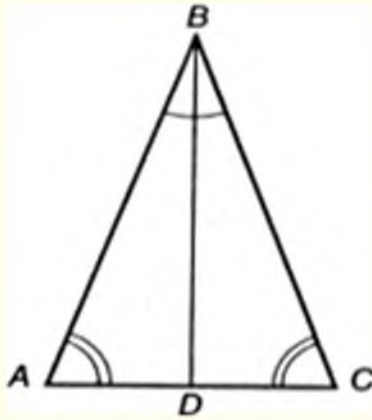
Рис. 10.1. Равнобедренный треугольник
