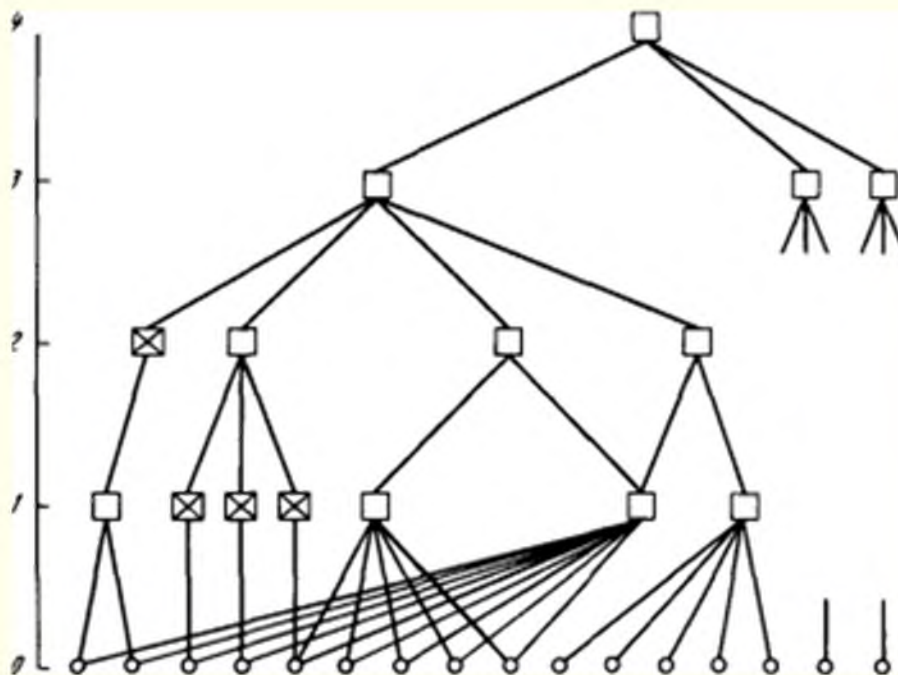
Рис. 2.2. Иерархия классификаторов
