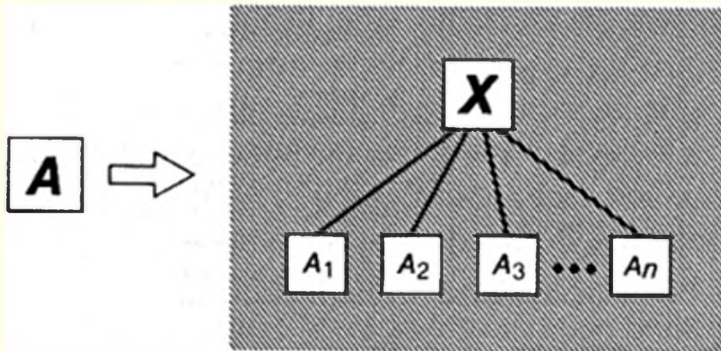
Рис. 3.1. Метасистемный переход
