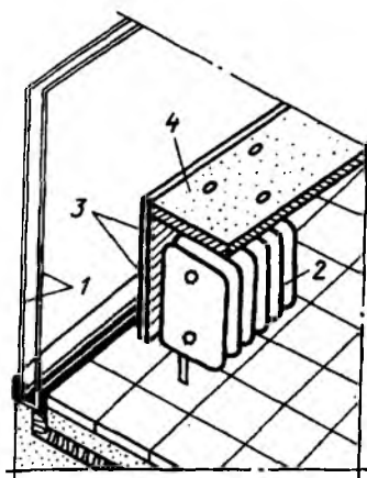
Рис. 6.32. Обдув стекла теплым воздухом, поднимающимся от радиатора, через отверстия в подоконной доске
