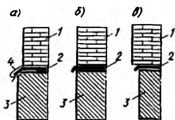
Рис. 8.18. Различные формы цоколя а — выступающий; б — в одной плоскости со стеной; в — западающий; 1 — наружная стена; 2 — гидроизоляция; 3 — цоколь; 4 — слив
