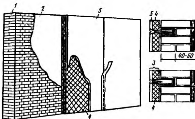
Рис. 5.32. Двуслойные плиты для утепления стен с наружной стороны 1 — оштукатуренная кирпичная стена; 2 — штукатурка; 3 — теплоизоляционная панель; 4 — минеральная вата; 5 — асбестоцементная облицовка
