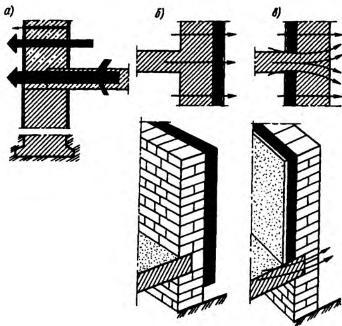
Рис. 8.41. Теплотери, происходящие через стену и через узел сопряжения балки перекрытия со стеной
