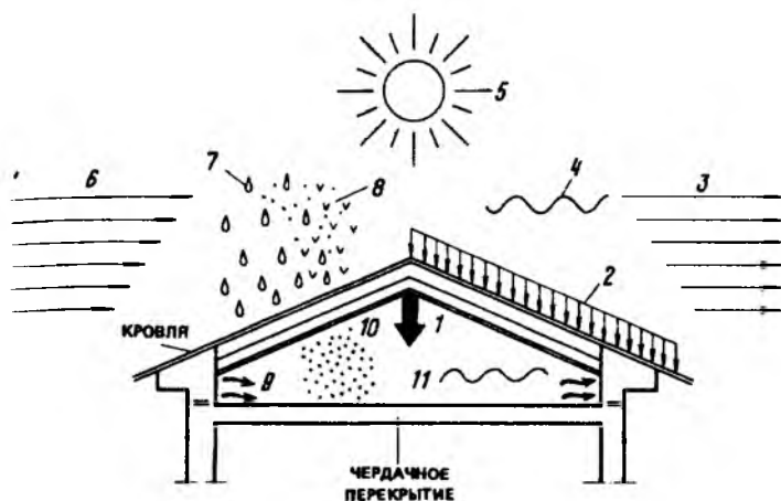
Рис. 7.1. Внешние воздействия на покрытие
