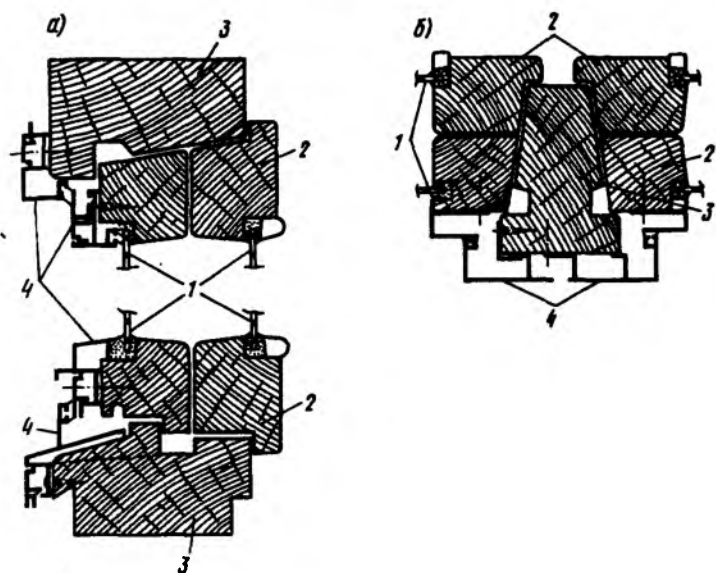
Рис. 6.2. Деревялоалюминиевый оконный блок с полной наружной облицовкой линейными элементами из алюминия a — вертикальный разрез; б — горизонтальный разрез; 1 — остекление; 2 — деревянный переплет; 3 — деревянная оконная коробка; 4 — алюминиевая облицовка;
