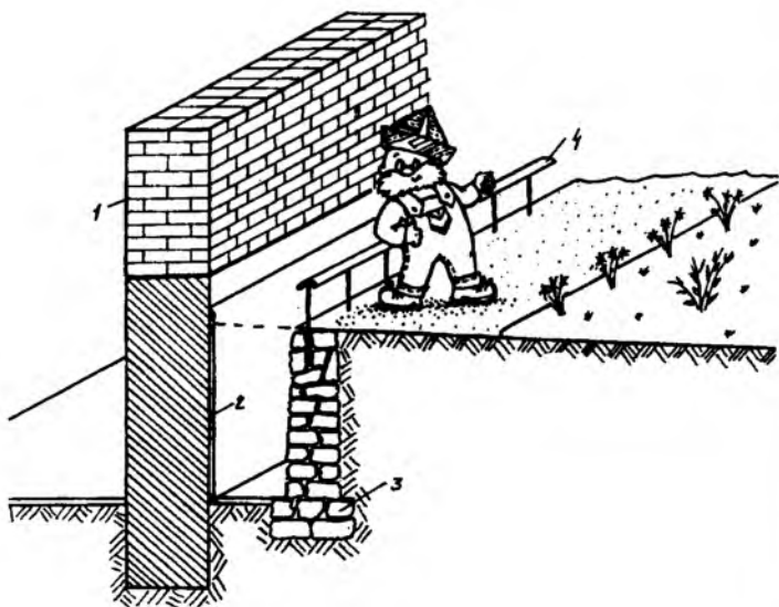
Рис. 8.32. Устройство водоотводной канавы с опорной стенкой 1 — стена; 2 — цементный раствор; 3 — опорная стенка; 4 — перила
