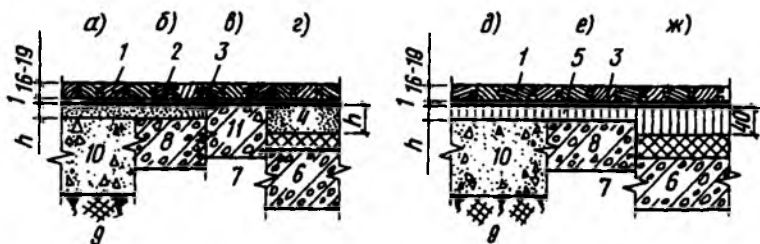
Рис. 8.29. Конструкции полов из штучного и наборного паркета а, д — по грунтовому основанию; б — по цементно-песчаной стяжке; в — по плите перекрытия; г, ж — с устройством тепло-, звукоизоляции; е — по стяжке из литого асфальтобетона; 1 — покрытие; 2 — цементно-песчаная стяжка; 3 — холодная водостойкая мастика; 4 — бетонная или цементно-песчаная стяжка; 5 — стяжка из литого асфальтобетона; 6 — плита перекрытия; 7 — тепло-, звукоизоляционный слой; 8 — плита перекрытия с неровной поверхностью; 9 — грунт основания; 10 — бетонный подстилающий слой; 11 — плита перекрытия с ровной поверхностью
