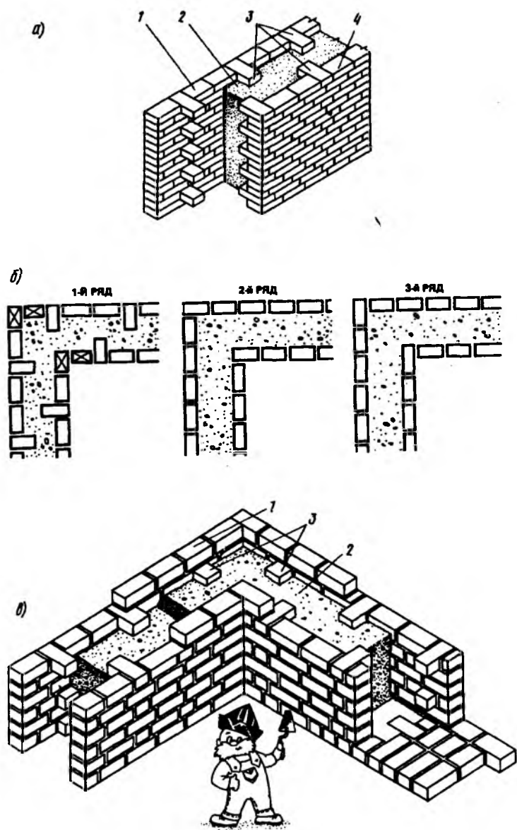
Рис. 5.15. Бетонно-анкерная кладка
