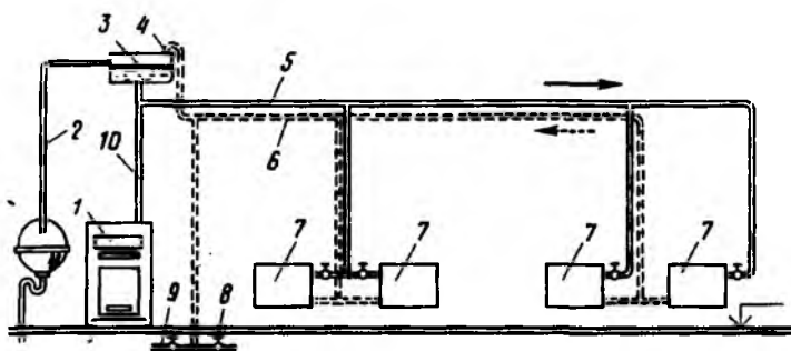
Рис. 9.11. Водяное отопление с прокладкой горячей и обратной линии под потолком
