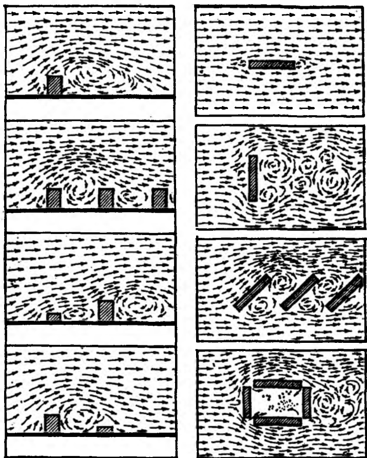
Рис. 1.3. Возникновение воздушных потоков в застройке различной конфигурации
