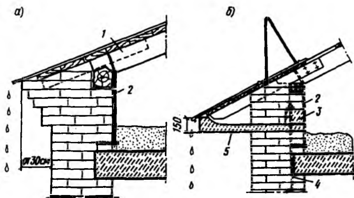
Рис. 2.23. Конструкции карнизов, защищающих стены от увлажнения дождем
