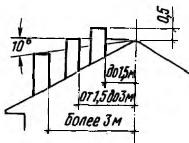
Рис. 9.2. Определение высоты трубы
