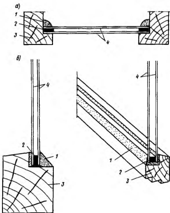
Рис. 6.20. Установка дополнительного стекла на картонную или резиновую прокладку
