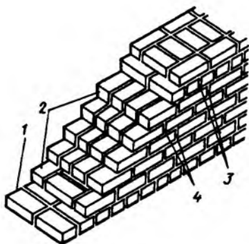
Рис. 5.9. Шестирядная система кладки
