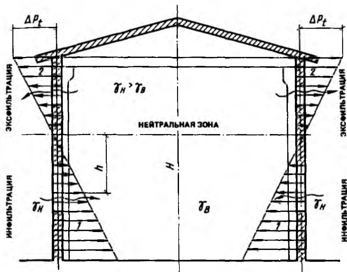
Рис. 6.5. Расположение нейтральной зоны при наличии теплового и ветрового напоров
