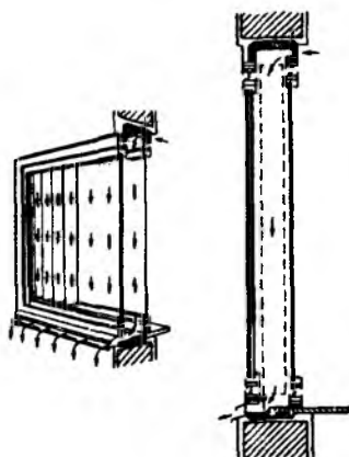
Рис. 6.31. Конструкция вентилируемого окна
