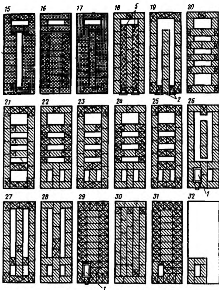
Рис. 9.7. Отопительная печь с теплоотдачей 4650 Вт
