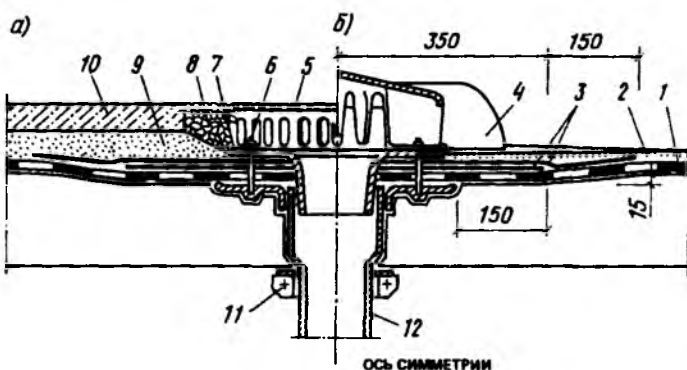
Рис. 7.11. Кровля в местах установки водосточных воронок
