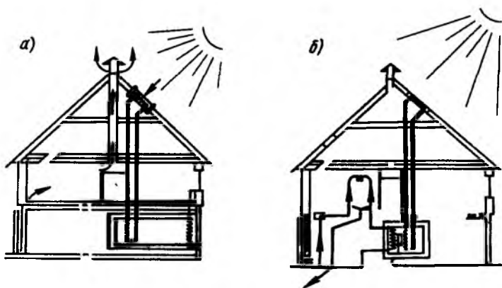
Рис. 10.10. Экспериментальный дом фирмы "PHILIPS" в Германии г. Аахен
