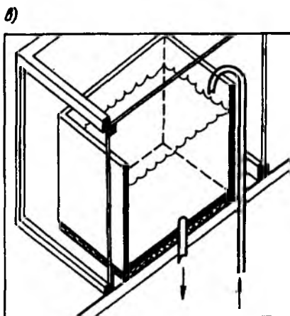
Рис. 10.3. Солнечная ловушка для нагрева воды
