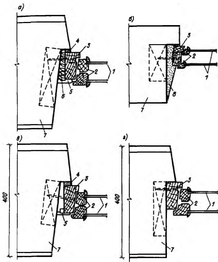
Рис. 6.7. Конструкции сопряжений оконных блоков с наружными стенами a — уплотнение зазора сухой антисептированной паклей (пенькой, очесами и др.); б — уплотнение зазора гипсоперлитовым раствором; в — сопряжение оконного блока со стеной без конопатки зазора; 2 — замоноличивание оконной коробки в стену; д — уплотнение зазора паклей, смоченной в цементном молоке; е — заделка зазора паклей и раствором гипсоцементно-пуццоланового вяжущего; ж — уплотнение зазора синтетическим жгутом; з — уплотнение зазора пенополиуретаном; 1 — остекление; 2 — переплет; 3 — оконная коробка; 4 — герметизирующая мастика; 5 — нащельник; 6 — сухая антисептированная пакля; 7 — наружная стена; 8 — гипсоперлитовый раствор; 9 — цементный раствор; 10 — пакля, смоченная в алебастровом или цементном растворах; 11 — раствор ГЦПВ; 12 — синтетический жгут
