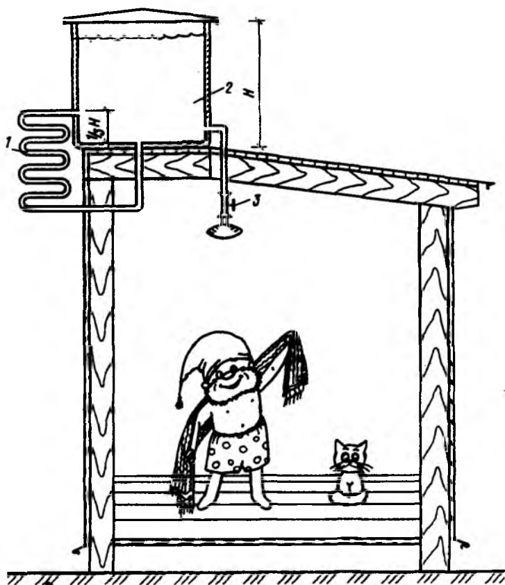
Рис. 10.4. Использование конденсатора от холодильника для нагрева воды солнечными лучами
