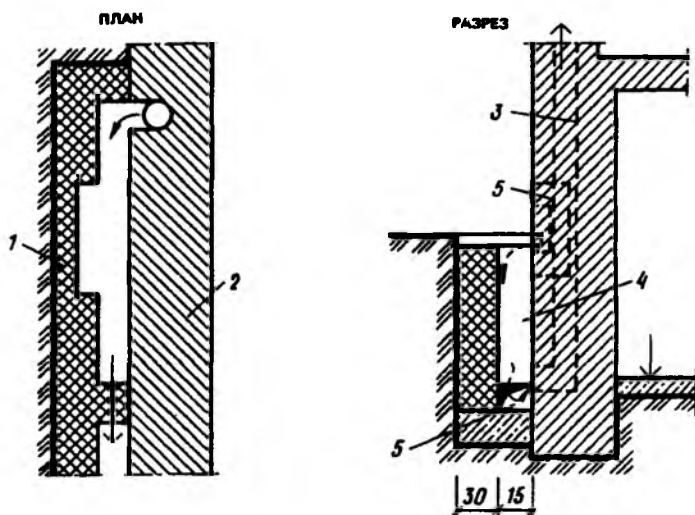
Рис. 8.34. Осушение подземной части стены путем устройства вентилируемой воздушной полости 1 — опорная стенка; 2 — осушаемая стена; 3 — вентиляционный канал; 4 — воздушная прослойка; 5 — вентиляционное отверстие
