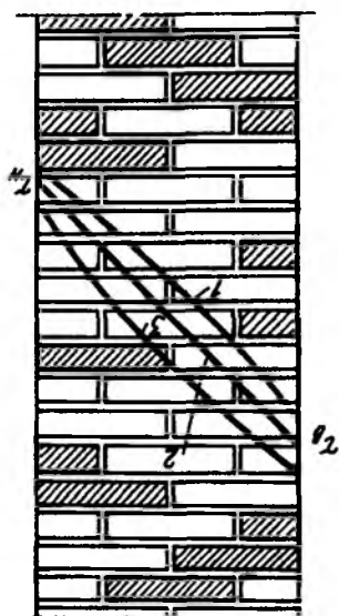
Рис. 2.13. Распределение температур в толще ограждения при инфильтрации (1), отсутствии воздухопроницаемости (2), эксфильтрации (3)
