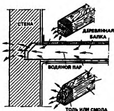
Рис. 8.22. Диффузия водяных паров в деревянной балке перекрытия
