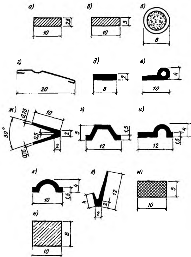
Рис. 6.14. Типы уплотняющих прокладок
