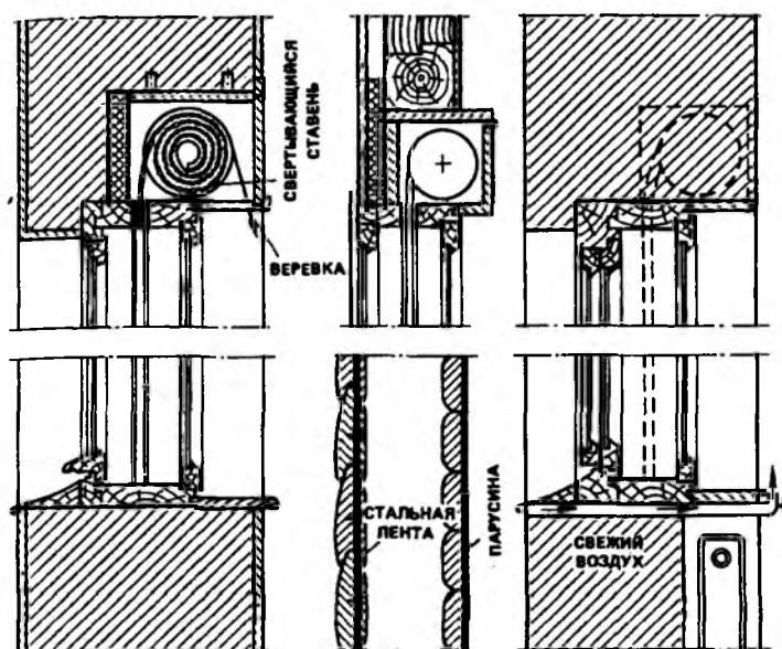
Рис. 6.25. Различные типы окон с экранами в межстекольном пространстве
