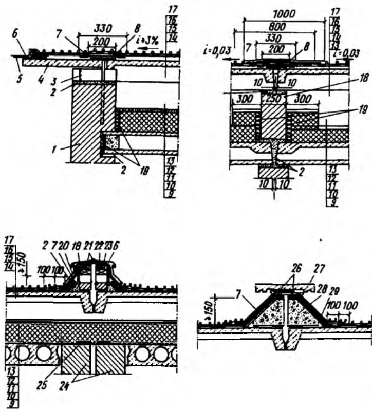
Рис. 7.6. Бесчердачная вентилируемая крыша
