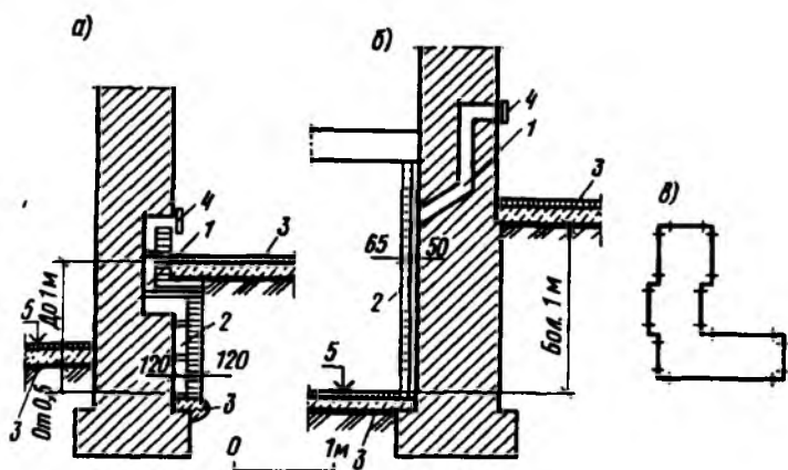
Рис. 8.35. Устройство вентилируемой полости с внутренней стороны подвала
