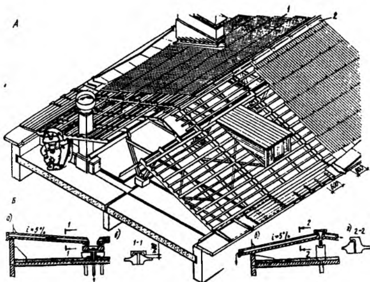
Рис. 7.12. Чердачные крыши
