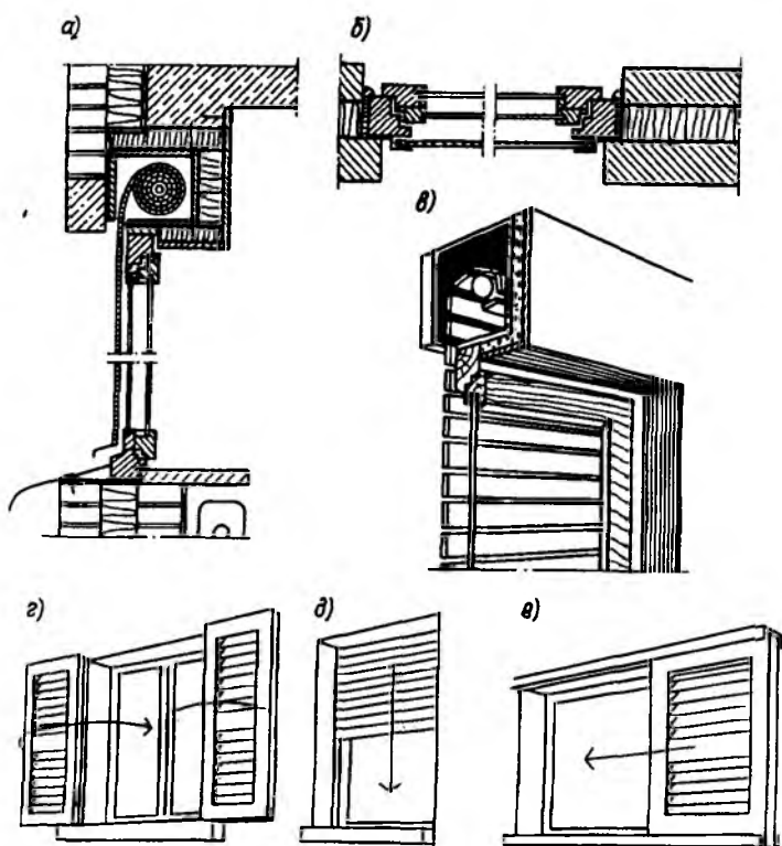
Рис. 6.22. Окна со свертывающимися экранами (а — вертикальный разрез; б — горизонтальный разрез; в — аксонометрия), закрывающимися ставнями (с); опускающимися жалюзи (д) и задвигающимися ставнями (е)
