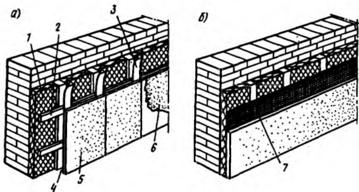
Рис. 5.26. Утепление кирпичной стены снаружи
