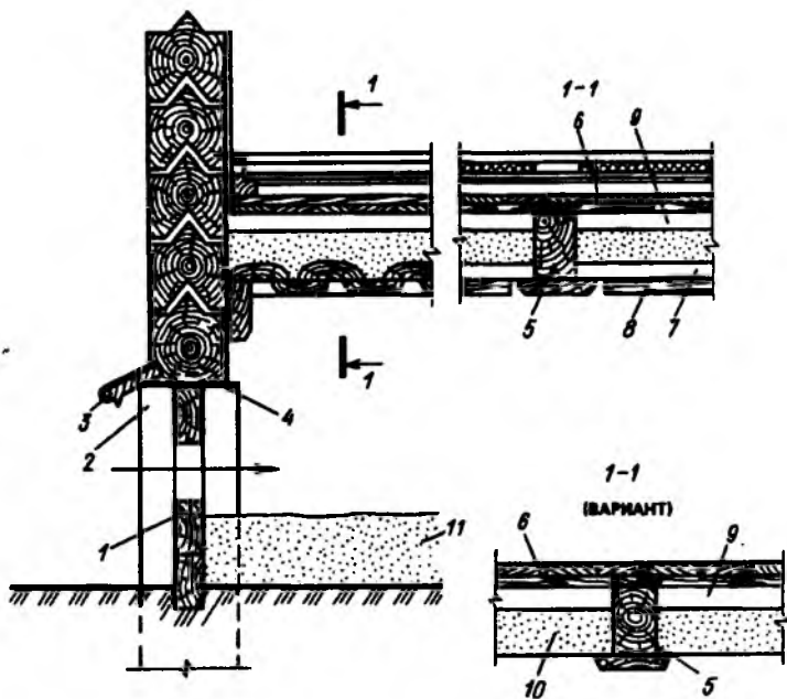
Рис. 8.14. Конструкция утепленного цокольного перекрытия с проветриваемым подпольем
