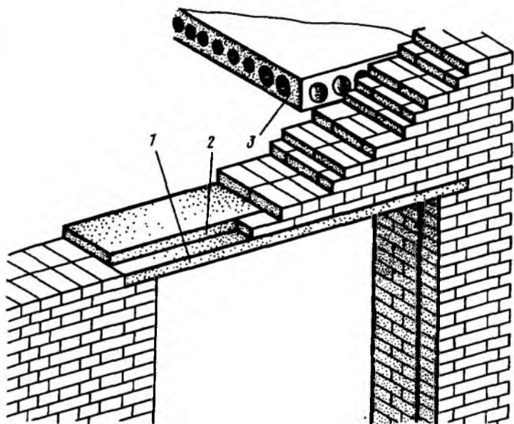
Рис. 5.35. Перекрытие проема железобетонными перемычками 1 — брусовая перемычка; 2 — плитная перемычка; 3 — плита перекрытия
