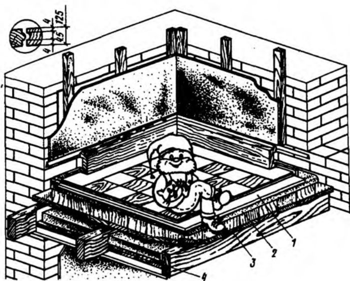
Рис. 8.1. Общий вид балочного перекрытия по деревянным балкам 1 — мастика; 2 — строительная бумага; 3 — дощатый настил; 4 — несущие деревянные балки
