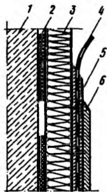
Рис. 5.29. Утепление стены плитами из пенопласта
