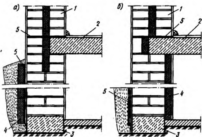
Рис. 8.38. Утепление стен подвалов пенопластом с наружной (а) и внутренней стороны (б)
