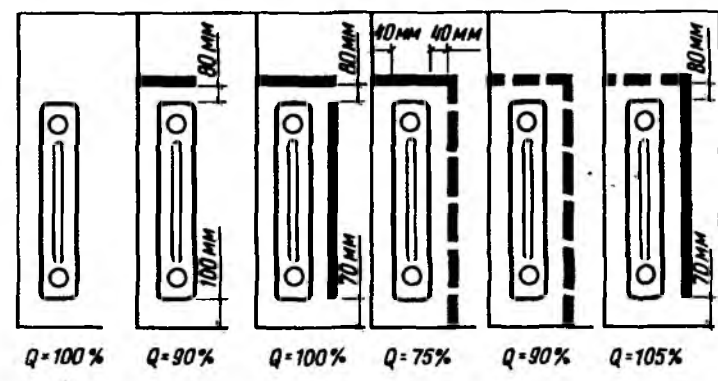
Рис. 9.15. Эффективность использования декоративных щитов около отопительных приборов
