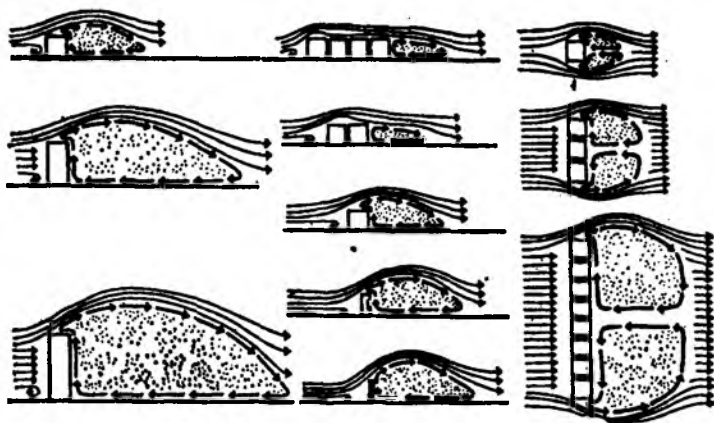
Рис. 1.4. Обтекание ветром группы зданий
