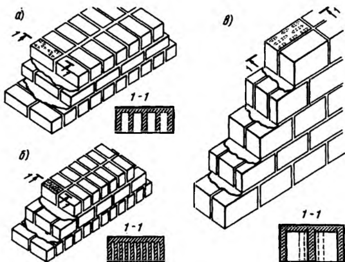
Рис. 5.11. Кладка из керамических камней (а), из утолщенного кирпича с пустотами (б), из бетонных камней
