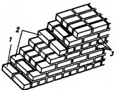
Рис. 5.10. Трехрядная система перевязки
