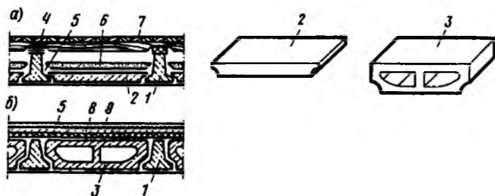
Рис. 8.3. Конструкция балочного перекрытия по железобетонным балкам a — с заполнением из плит; б — с заполнением из пустотелых блоков; 1 — балки; 2 — плиты; 3 — пустотелые блоки; 4 — изоляция ударного шума (упругие прокладки); 5 — промазка щелей раствором или подстилка толя; 6 — усиление изоляции воздушного шума (песок); 7 — пол по лагам; 8 — изоляция воздушного и ударного шумов; 9 — пол по стяжке
