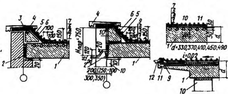
Рис. 7.7. Бесчердачная крыша из легкбетонных панелей
