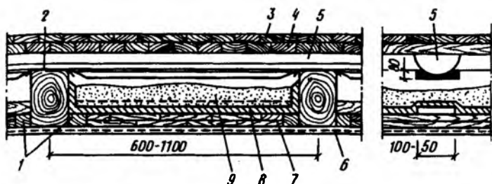
Рис. 8.5. Перекрытие по брусчатым балкам
