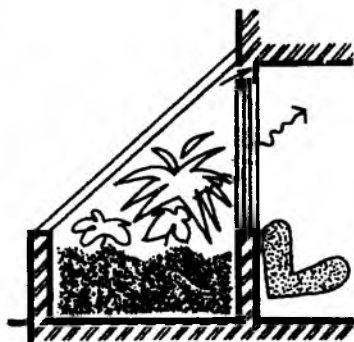
Рис. 10.9. "Зимний сад" у южной стены дома
