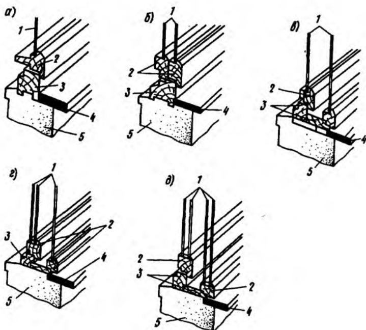
Рис. 6.1. Различные конструкции деревянных оконных блоков, применяемых в домах
