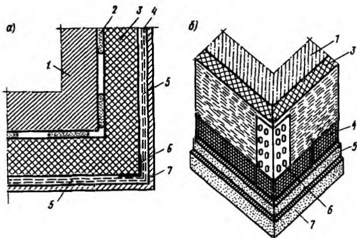
Рис. 5.34. Конструктивное решение утепления угла а — план; б — аксонометрия; 1 — стена; 2 — клеящая мастика; 3 — утеплитель (пенопласт); 4 — сетка; 5 — выравнивающий слой; 6 — алюминиевые уголок; 7 — отделочный слой
