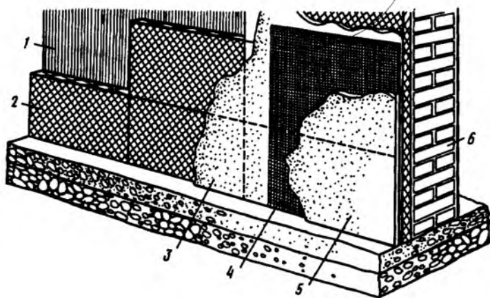
Рис. 5.30. Утепление стен по существующей штукатурке теплоизоляционными плитками
