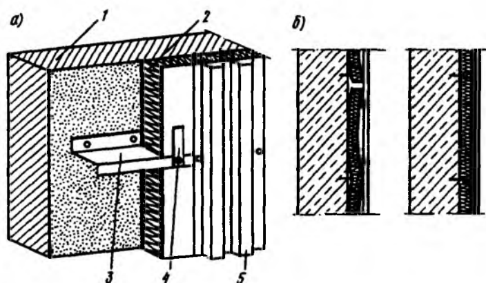
Рис. 5.28. Крепление утеплителя из минераловатных плит к бетонной стене
