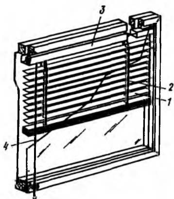
Рис. 6.26. Межстекольная штора-жалюзи
