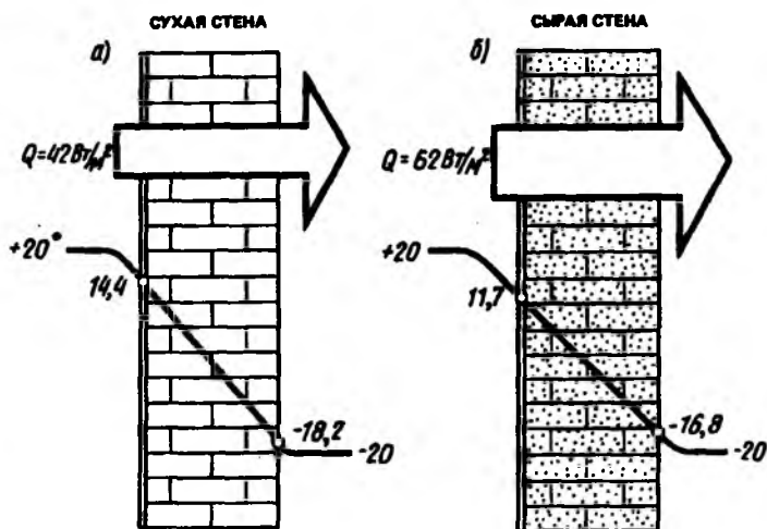
Рис. 2.5. Влияние влажности материала на теплозащитные свойства кирпичной стены
