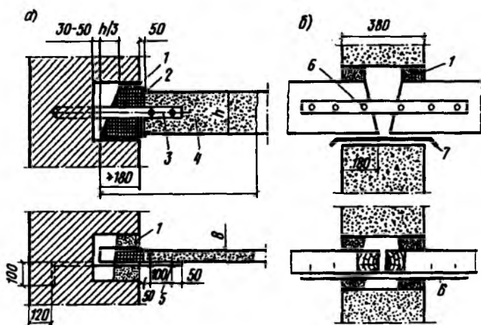
Рис. 8.23. Опираие деревянных балок на каменные стены a — одной балки; б — двух балок: 1 — заделка раствором; 2 — два слоя толя на смоле; 3 — анкер; 4 — антисептированная часть балки; 5 — гвоздь; 6 — стальная накладка размером 50х6 мм; 7 — два слоя толя
