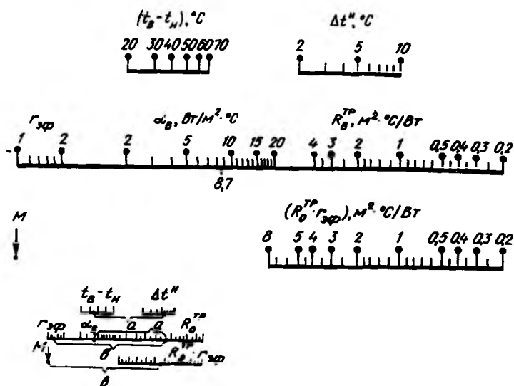
Рис. 11.1. Номограмма для определения требуемого сопротивления теплопередаче
