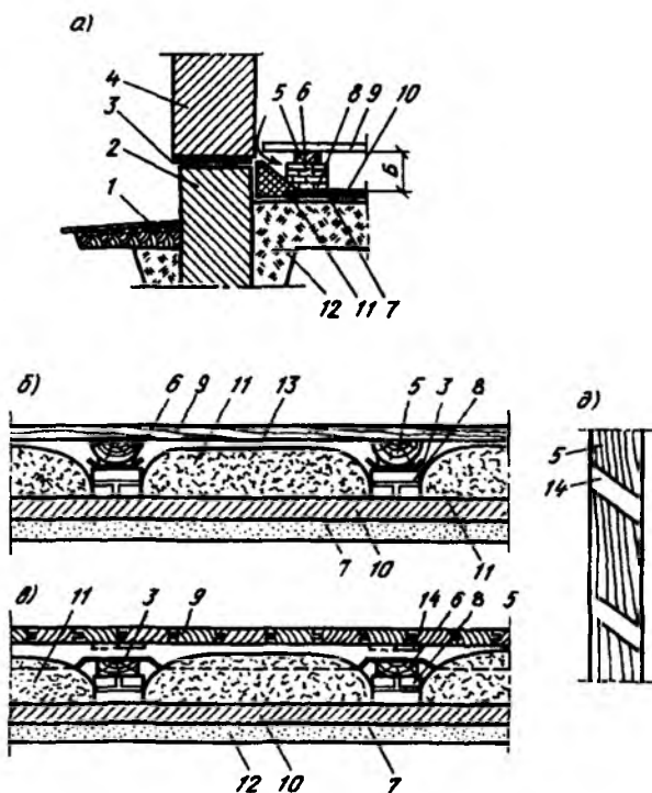
Рис. 8.13. Конструкции перекрытий над теплым подпольем
