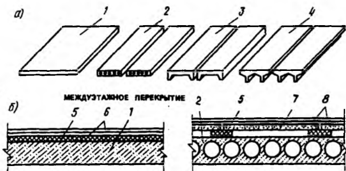
Рис. 8.27. Перекрытия по железобетонным плитам
