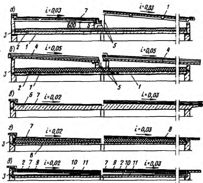
Рис. 7.5. Принципиальные схемы конструкций бесчердачных железобетонных крыш
