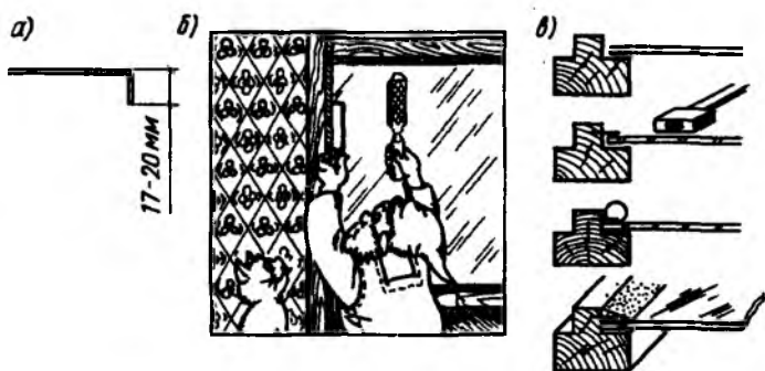
Рис. 6.9. Вставка стекол на одинарной замазке а — проволочная шпилька; б — закрепление стекла проволочными шпильками стамеской; в — последовательность операции
