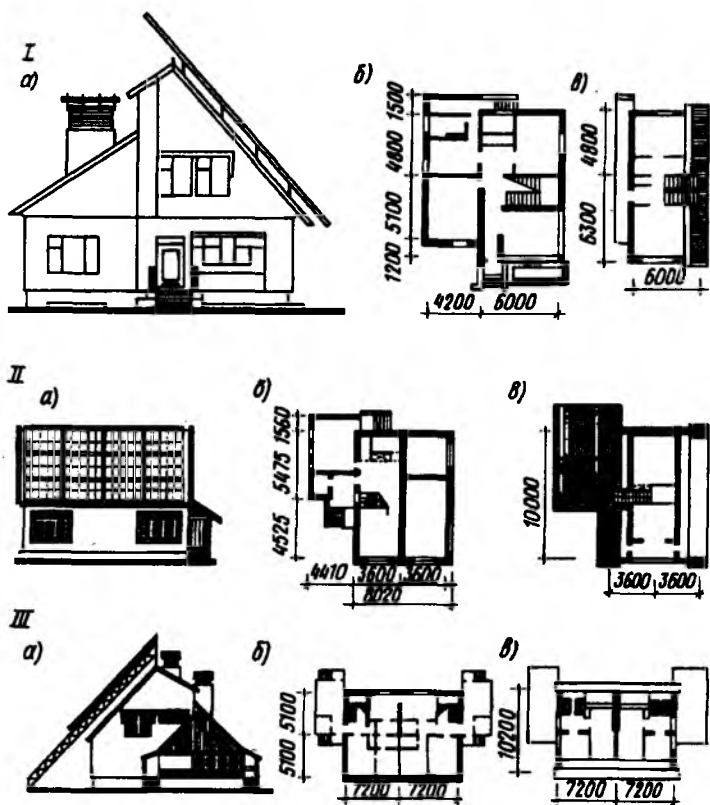
Рис. 10.2. Солнечные коллекторы на крыше мансардного одноквартирного (I) и двухквартирного домов (II, III) а — общий вид; б, в — планы этажей
