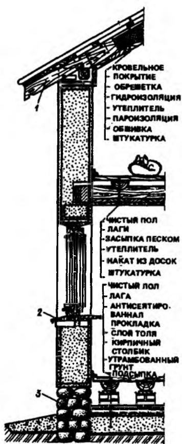
Рис. 5.20. Монолитные стены из легкого бетона
