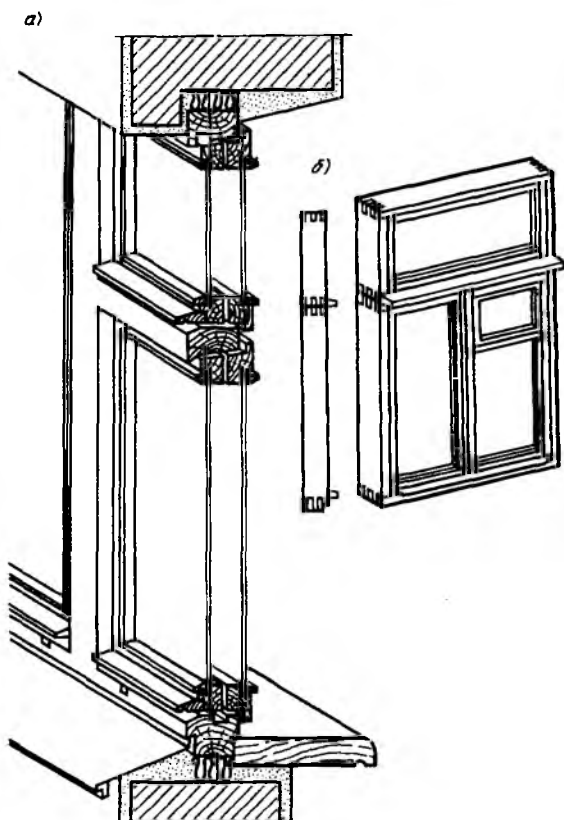
Ри. 6.6. Установка оконных блоков в проем
