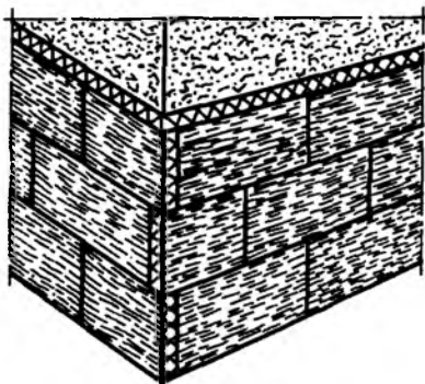
Рис. 5.33. Расположение плит утеплителя с наружной стороны угла
