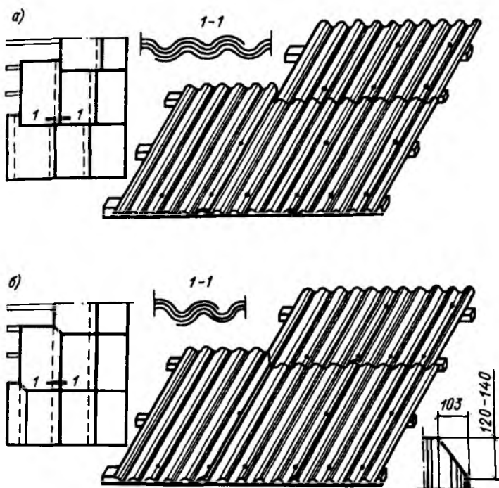
Рис. 7.16. Покрытие крыши
