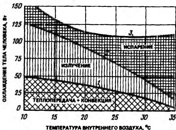
Рис. 2.7. Потери тепла человеком, не производящим физической работы 1 — вследствие теплопередачи и конвекции; 2 — вследствие теплопередачи, конвекции и излучения; 3 — вследствие теплопередачи, конвекции, излучения и испарения
