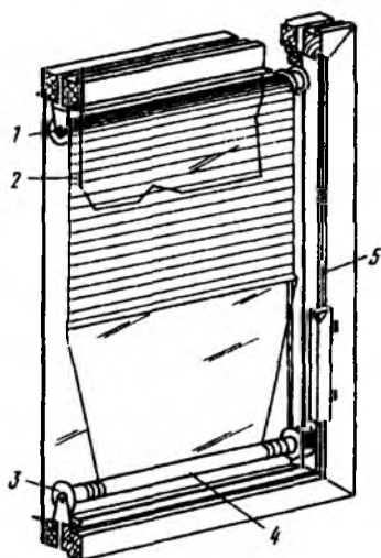
Рис. 6.29. Штора с комбинированным экраном 1 — верхний барабан; 2 — полотно из полупрозрачной ткани или металлизированной пленки; 3 — нижний барабан; 4 — непрозрачное темное полотно; 5 — шнур
