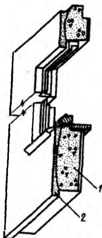
Рис. 5.18. Однослойная бетонная панель наружных стен 1 — конструктивно-теплоизоляционный бетон; 2 — защитно-отделочный слой
