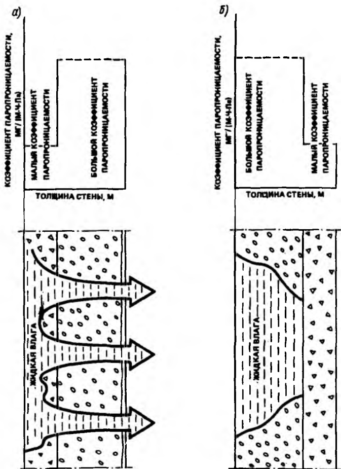
Рис. 2.17. Условия высыхания и отсыревания конструкций двухслойной наружной стены
