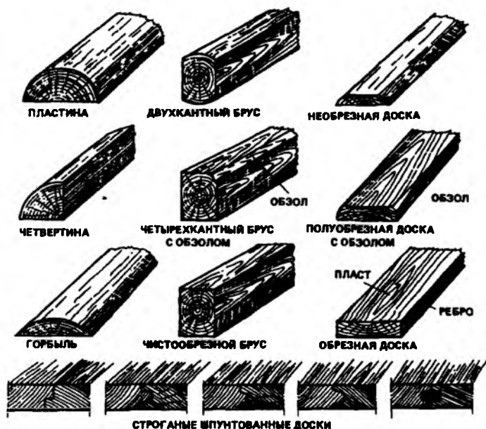
Рис. 4.2. Пиломатериалы, используемые в строительстве
