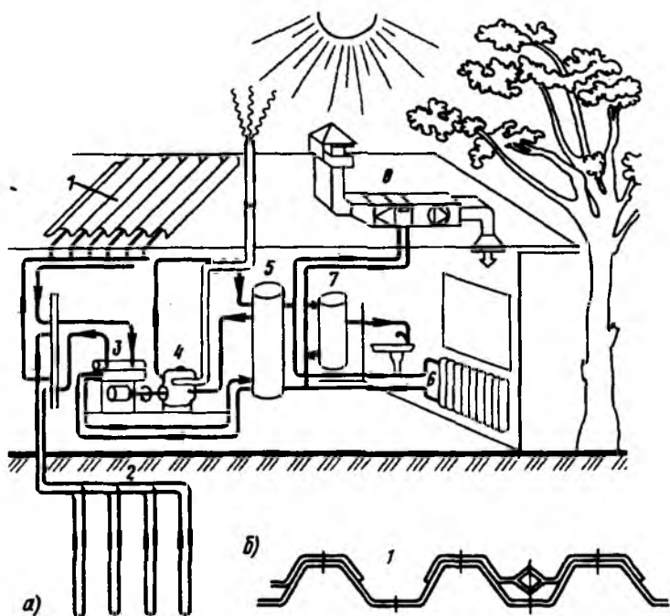
Рис. 10.11. Тепловая установка здания гимназии в Швеции г. Кунгсбака a — общая схема; б — поперечный разрез кровельного настила; 1 — солнечный коллектор; 2 — грунтовой аккумулятор тепла; 3 — тепловой насос; 4 — дизельный двигатель; 5 — резервуар для воды; 6 — радиатор; 7 — водонагреватель; 8 — вентиляционная установка с теплообменником
