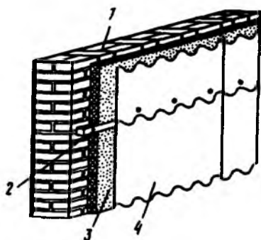
Рис. 5.27. Утепление минераловатными плитами
