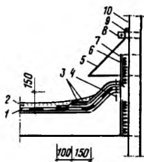
Рис. 7.10. Пропуски труб
