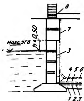
Рис. 8.17. Гидроизоляция подвала при больших напорах грунтовых вод, устраиваемая по внутренней поверхности стен 1 — бетонная подготовка; 2 — цементная стяжка; 3 — рулонная изоляция; 4 — цементный слой; 5 — железобетонная коробчатая конструкция; 6 — чистый пол; 7 — цементная штукатурка по битумной обмазке; 8 — гидроизоляция
