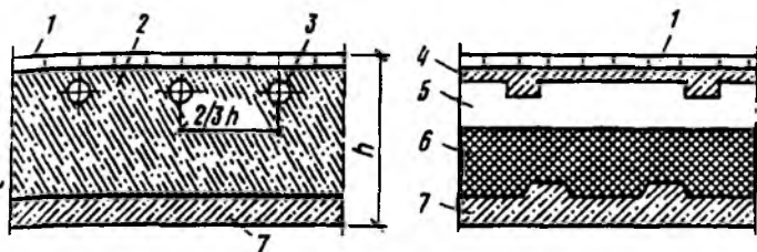
Рис. 7.3. Бесчердачные покрытия с вентилируемыми каналами 1 — кровля; 2 — легкий бетон; 3 — вентилируемые цилиндрические каналы; 4 — железобетонная плита; 5 — вентилируемая воздушная прослойка; 6 — утеплитель; 7 — несущая железобетонная плита
