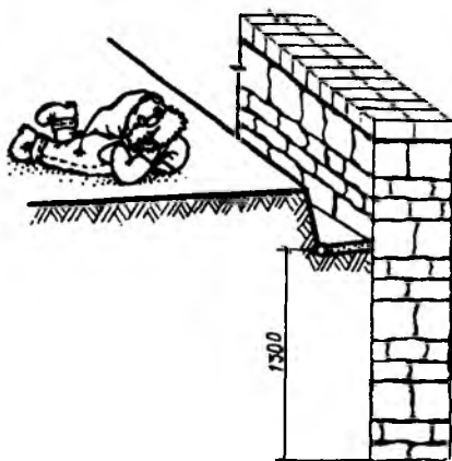
Рис. 8.30. Устройство водоотводной канавы вокруг дома
