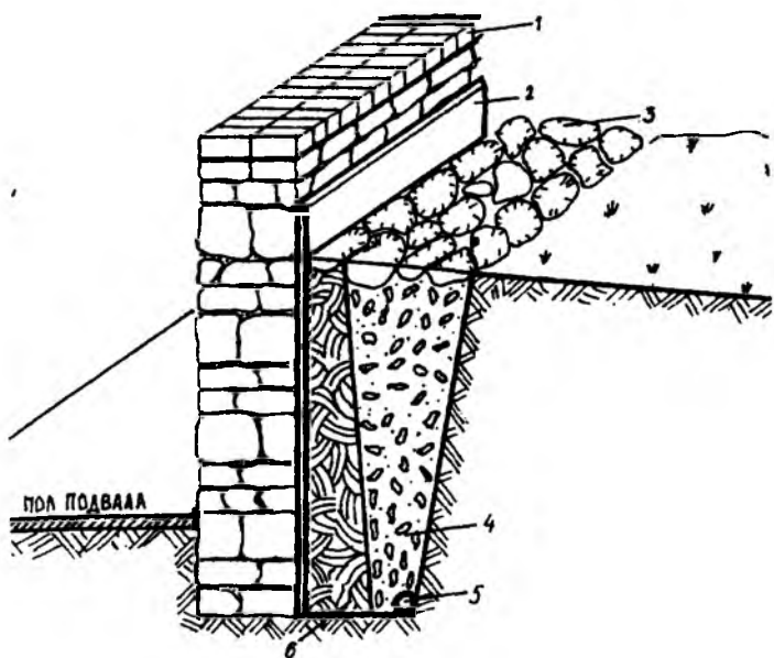
Рис. 8.33. Дренаж вдоль дома
