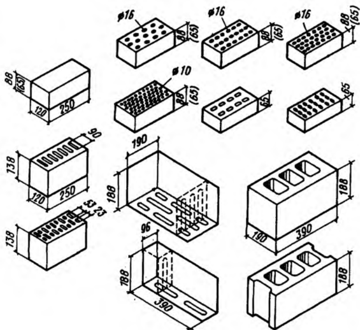
Рис. 4.1. Виды кирпича и керамических камней, используемых в строительстве
