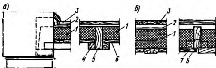
Рис. 8.9. Цокольное перекрытие с черным полом, уложенным по черепным брускам (а) и с черным полом, подшитым снизу балками (б) 1 — утеплитель; 2 — пароизоляция; 3 — доски пола; 4 — черепной брусок; 5 — балки; 6 — черный пол; 7 — подшивка
