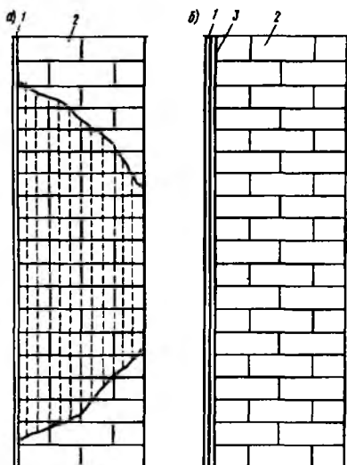
Рис. 2.16. Влияние пароизоляции на внутренней поверхности стены из силикатного кирпича на ее влажностной режим
