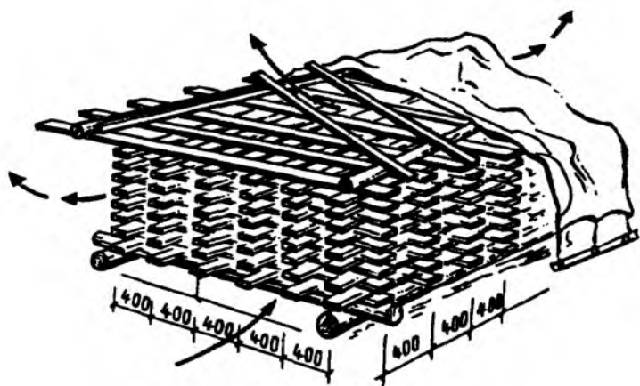
Рис. 4.3. Укладка пиломатериалов в штабель
