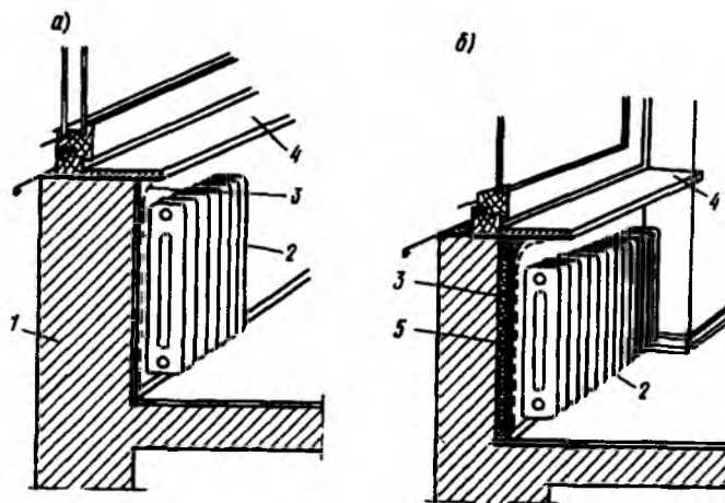
Рис. 9.14. Утепление стены за отопительным прибором путем установки блестящей алюминиевой фольги на внутренней поверхности стены (а) или установкой теплоизоляционного материала, с покрытием его алюминиевой фольгой (б) 1 — наружная стена; 2 — радиатор; 3 — алюминиевая фольга; 4 — подоконник; 5 — утеплитель
