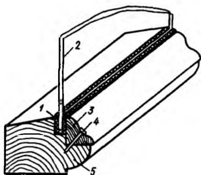
Рис. 6.12. Вставка стекла на резиновой прокладке
