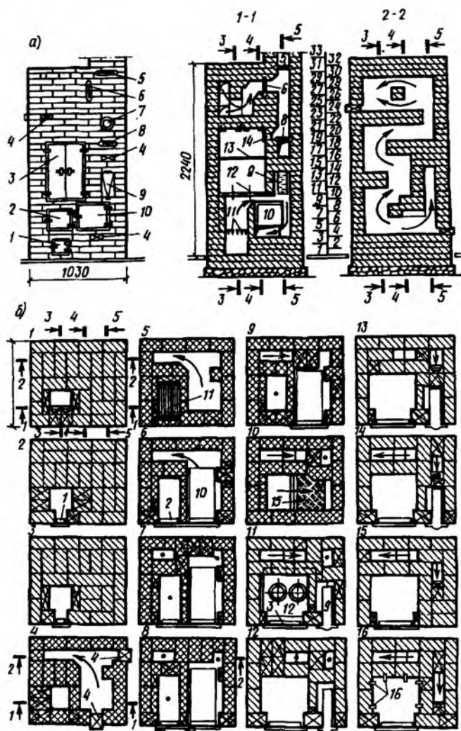
Рис. 9.8. Отопительно-варочная печь типа "шведка"
