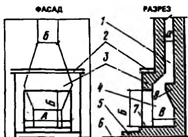
Рис. 9.19. Камин 1 — дымоборник; 2 — каминная доска; 3 — портал камина; 4 — топливник; 5 — подиум; 6 — предтопочный лист; 7 — под камин; 8 — дымовой уступ; А — ширина портала; В — высотв портала; В — глубина топливника; а — ширина дымохода
