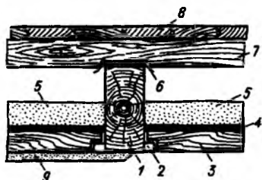
Рис. 8.2. Конструкция балочного перекрытия по деревянным балкам с накатом
