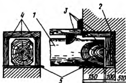
Рис. 8.24. Открытая заделка концов балки в стену толщиной 0,51 м 1 — балка; 2 — утеплитель; 3 — деревянная доска; 4 — деревянный короб; 5 — прокладка из толя в один-два слоя
