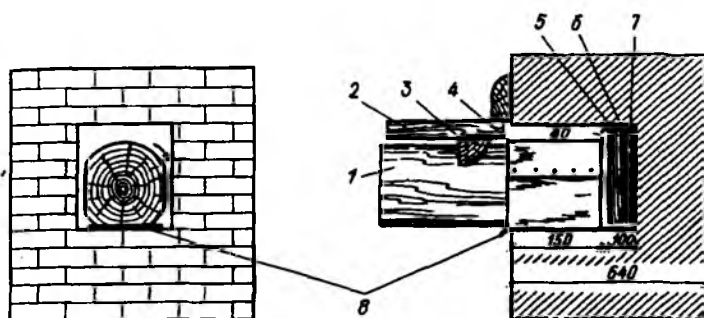
Рис. 8.25. Заделка концов балки в стену толщиной 0,64 см и более 1 — балка; 2 — пол; 3 — лага; 4 — обернутый двумя слоями толя или рубероида конец балки; 5 — доска толщиной 25 мм; 6 — толь; 7 — утеплитель — один слой войлока; 8 — толь или рубероид в один-два слоя
