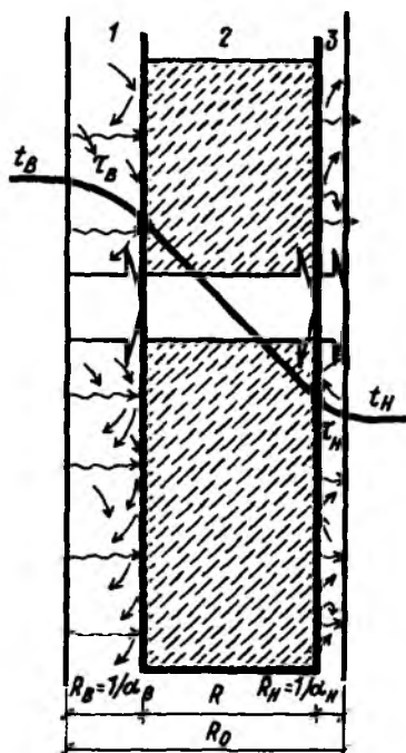
Рис. 2.6. Сопротивление теплопередаче стены
