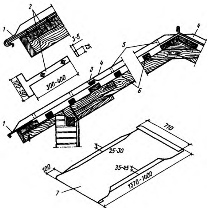
Рис. 7.15. Детали кровли из стальных листов
