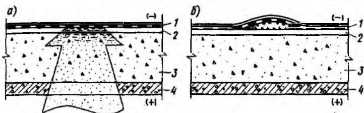
Рис. 7.4. Образование льда под кровельным ковром бесчердачного покрытия а — проникновение водяных паров из внутреннего помещения через бесчердачное перекрытие и их конденсация под гидроизоляционным ковром; б — отрыв гидроизоляционного ковра от перекрытия в результате расширения замерзшей воды; 1 — кровля; 2 — стяжка; 3 — керамзитобетонные плиты; 4 — железобетонные плиты
