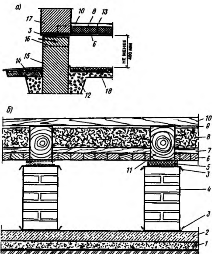
Рис. 8.11. Конструкция холодного подполья
