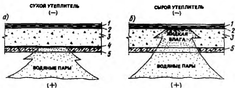
Рис. 2.19. Проникновение водяных паров в конструкцию бесчердачного перекрытия при устройстве пароизоляции (а) и без нее (б) 1 — кровля; 2 — стяжка; 3 — теплоизоляция; 4 — пароизоляция; 5 — железобетонная плита
