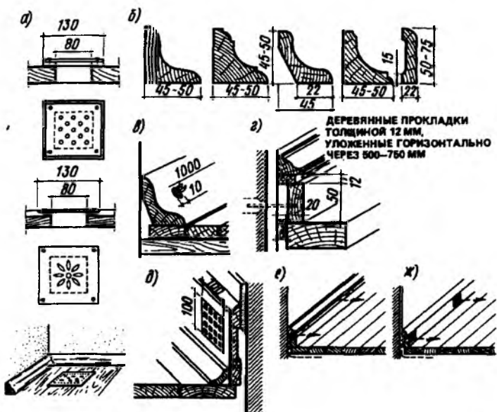
Рис. 8.10. Устройства для проветривания подполья
