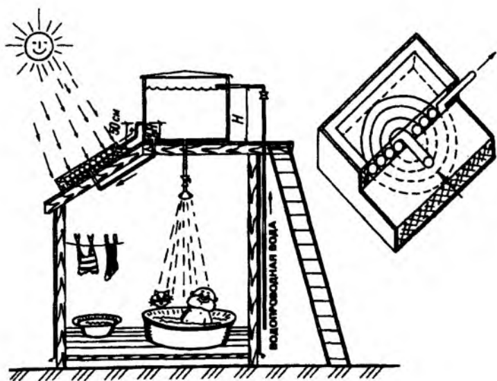
Рис. 10.5. Использование резинового шланга, свернутого кольцами, для нагрева воды
