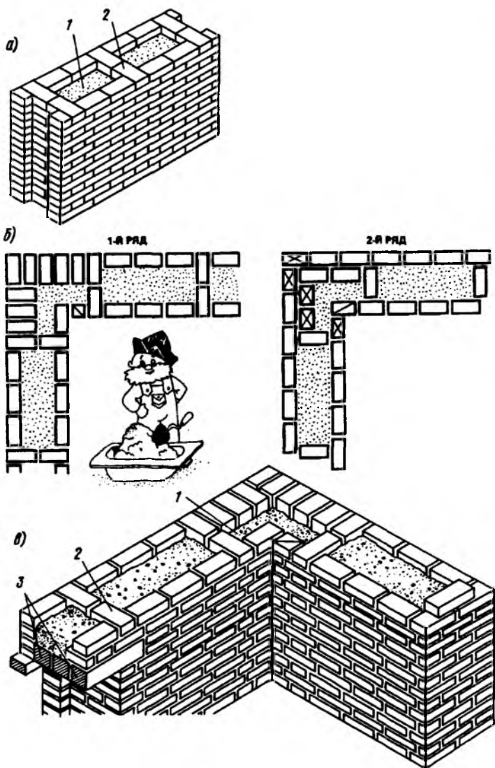
Рис. 5.14. Колодцевая кладка
