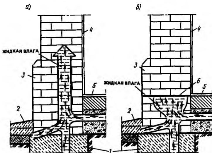
Рис. 2.21. Увлажнение конструкции цокольного узла без гидроизоляции (а) и с гидроизоляцией (б)
