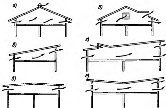
Рис. 7.2. Вентиляция чердачного пространства
