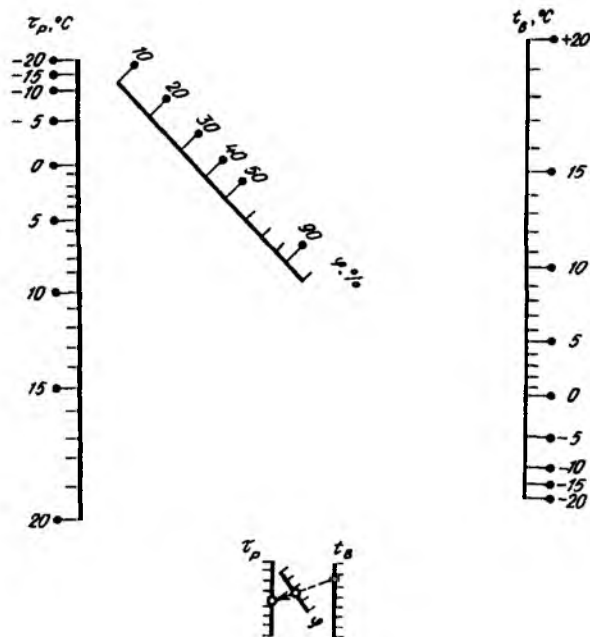
Рис. 11.13. Номограмма для определения температуры точки росы
