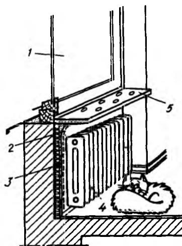
Рис. 6.33. Утепление радиаторной стенки с установкой отражающего экрана из алюминиевой фольги и обдув стекла теплым воздухом через отверстия в подоконнике
