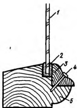
Рис. 6.11. Вставка стекла на штапиках
