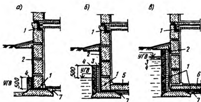
Рис. 8.16. Гидроизоляция подвалов
