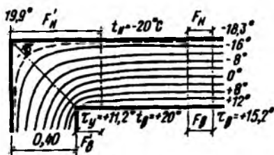
Рис. 3.2. Понижение температуры внутренней поверхности угла
