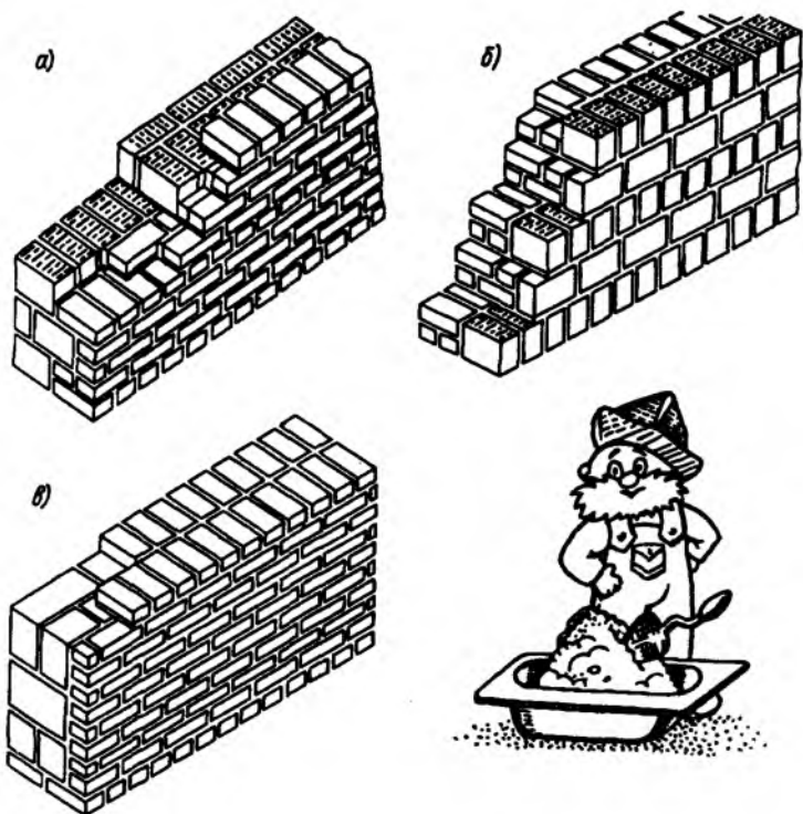
Рис. 5.12. Смешанная кладка
