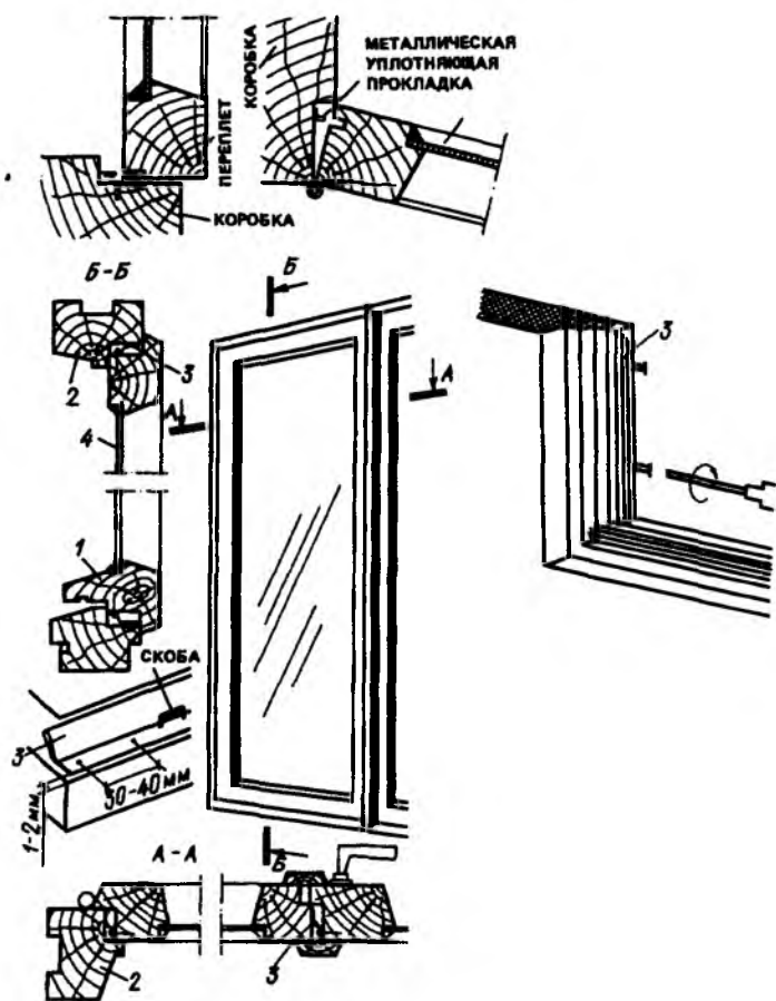
Рис. 6.17. Повышение герметичности окон установкой металлической ленты
