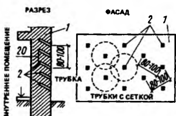
Рис. 8.36. Устройство осушающих каналов в стене с наружной стороны 1 — осушаемая стена; 2 — каналы
