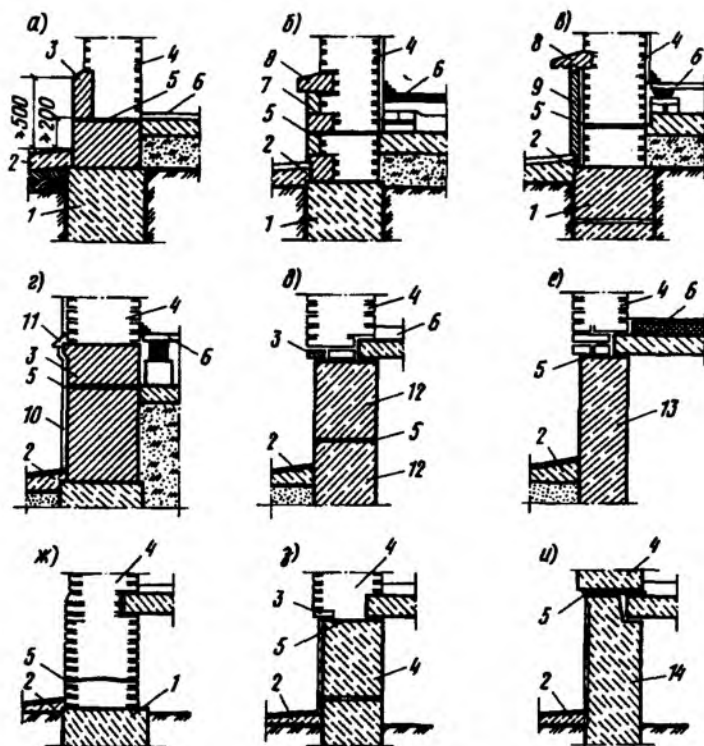
Рис. 8.19. Конструкция цоколя
