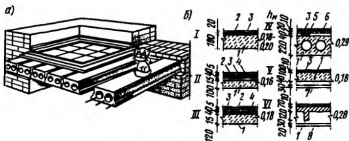
Рис. 8.4. Конструкция плитного перекрытия a — общий вид плитного перекрытия; б — конструктивные схемы плитных перекрытий; 1 — панель перекрытия; 2 — упругая прокладка; 3 — пол; 4 — железобетонная или бетонная плита пола; 5 — лаги; 6 — черный пол; 7 — потолок самонесущий; 8 — потолок подвесной; I—III — варианты плитных покрытий
