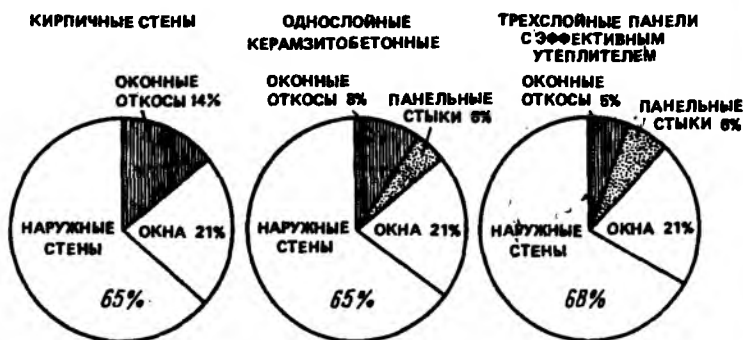
Рис. 2.12. Площади различных элементов наружных ограждений и теплотери
