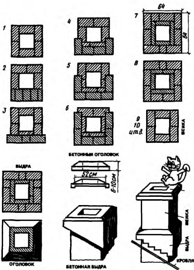
Рис. 9.4. Кладка выдры, шейки и оголовка трубы 1—10 — ряды кладки
