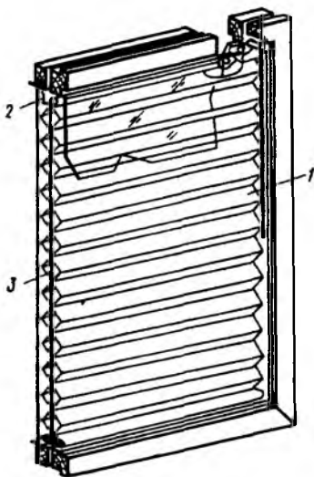
Рис. 6.30. Штора с объемным экраном 1 — экран из складчатых полотен; 2 — планка; 3 — шнур
