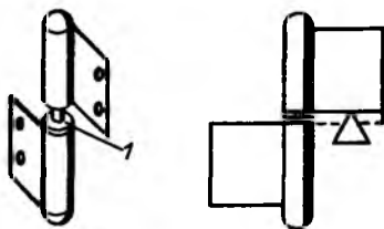
Рис. 6.18. Регулирование высоты подвески оконной рамы установкой на петле проволочного кольца
