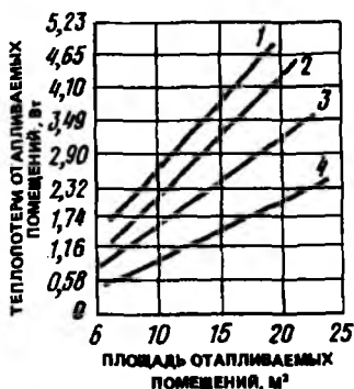
Рис. 9.17. График для определения ориентировочных теплопотерь одноэтажного дома 1 — прихожая; 2 — помещения с двумя углами; 3 — помещения с одним углом; 4 — неугловое помещение
