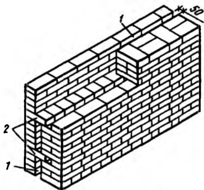
Рис. 5.16. Кладка с воздушной прослойкой
