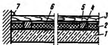
Рис. 8.39. Утепление перекрытий (дощатыми полами по деревянным лагам, засыпным утеплителем или минеральной ватой
