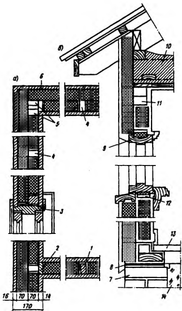
Рис. 5.5. Детали конструкций каркасного дома с утеплением стен фибролитовыми плитами
