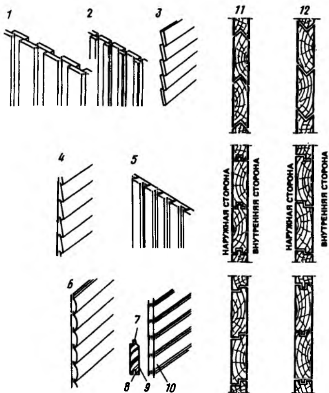
Рис. 5.6. Варианты облицовки фасада досками
