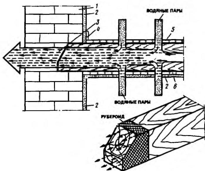
Рис. 2.20. Диффузия водяного пара в деревянной потолочной балке 1 — кирпичная стена; 2 — слой штукатурки; 3 — воздушный зазор между торцом деревянной потолочной балки и кирпичом; 4 — плинтус; 5 — пол из шпунтованных досок; 6 — доски
