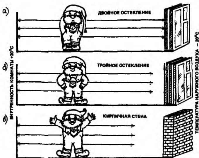
Рис. 3.4. Потери тепла с поверхности тела человека при теплообмене излучением с внутренними поверхностями комнаты (левая сторона рисунков) и с двойным (а), с тройным (б) остеклением и с наружной кирпичной стеной (в) (правая сторона рисунков)
