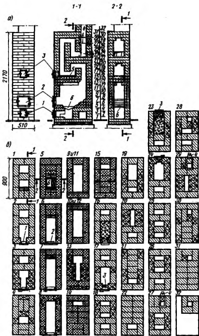
Рис. 9.6. Отопительная печь с теплоотдачей 2200 Вт
