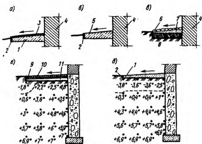
Рис. 8.21. Отмостки
