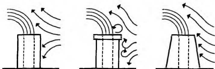
Рис. 9.3. Различные конфигурации труб
