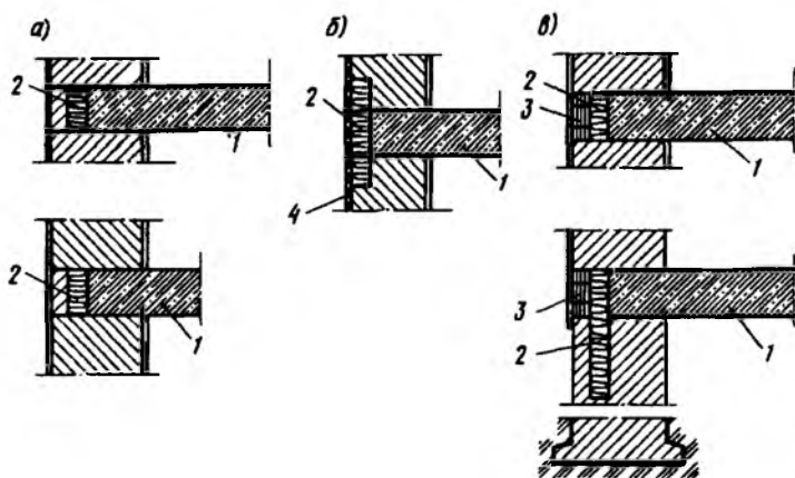
Рис. 8.42. Утепление узла сопряжения железобетонной балки с наружной стеной
