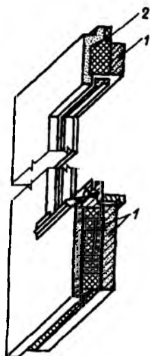
Рис. 5.19. Трехслойная панель 1 — конструктивный бетон; 2 — эффективный утеплитель
