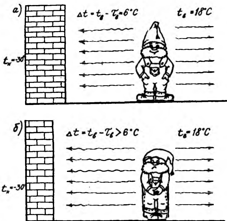
Рис. 2.10. Потеря тепла излучением при теплообмене человека с внутренней частью комнаты (правая сторона рисунка) и с наружной стеной (левая сторона рисунка)
