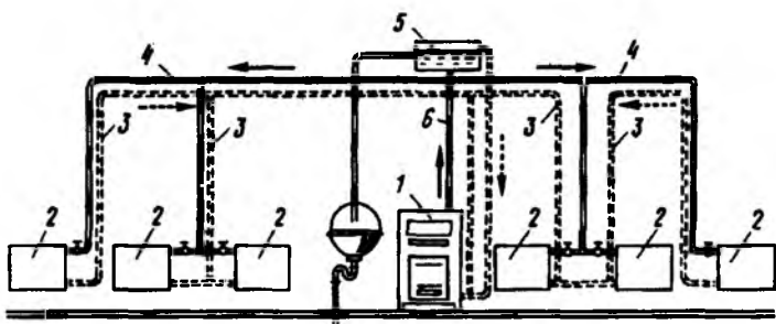
Рис. 9.12. Водяное отопление с прокладкой горячей и обратной линии под приборами 1 — котел; 2 — отопительные приборы; 3 — обратная линия; 4 — горячая разводящая линия; 5 — расширительный бак; 6 — главный стояк
