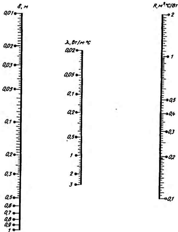
Рис. 11.2. Номограмма для определения толщины конструкции
