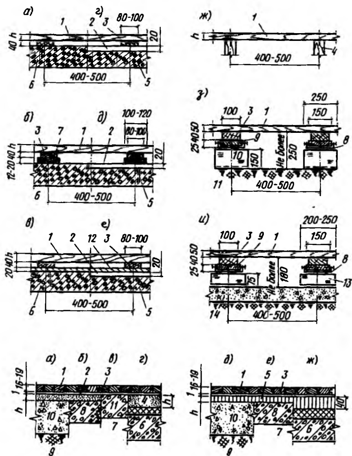
Рис. 8.28. Конструкции деревянных полов из досок или паркетных досок и щитов или древесно-стружечных плит для полов
