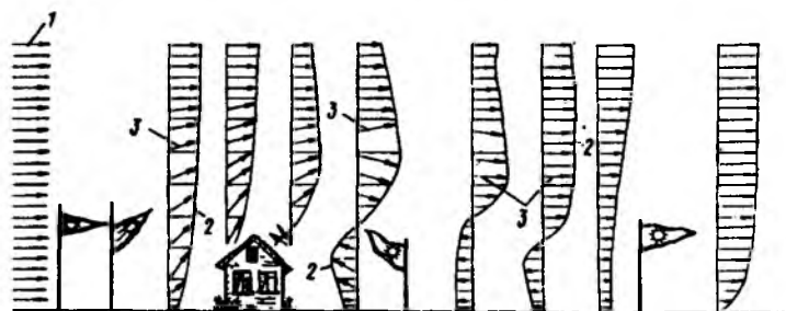
Рис. 1.1. Обтекание ветром прямоугольного здания 1 — ветер; 2 — эпюра давления от ветра; 3 — направленные движения ветровых потоков
