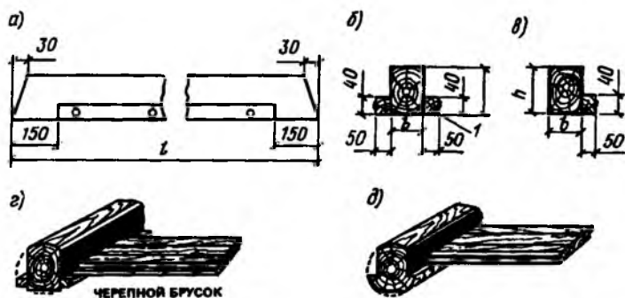
Рис. 8.6. Деревянная балка с черепными брусками
