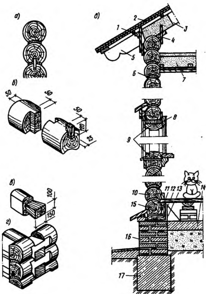
Рис. 5.2. Конструкции наружных рубленых стен
