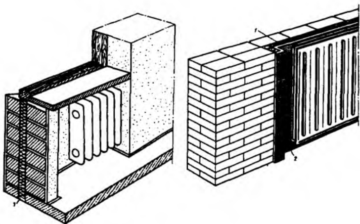
Рис. 5.25. Утепление стены за радиатором 1 — утепляющий материал; 2 — алюминиевая фольга
