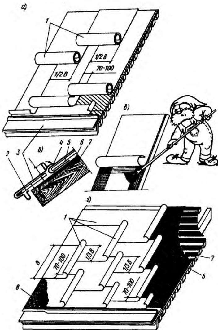
Рис. 7.14. Кровля из рулонных материалов
