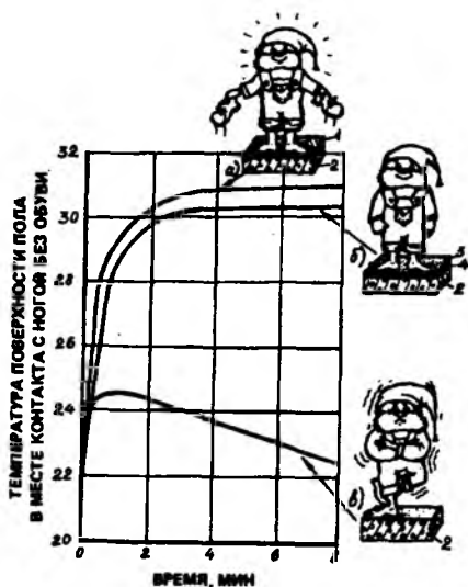
Рис. 2.11. Тепловое ощущение человека от теплого (а, б) и холодного полов (в) 1 — паркет толщиной 16 мм; 2 — перекрытие; 3 — линолеум толщиной 4 мм; 4 — теплозвукоизоляционная подоснова
