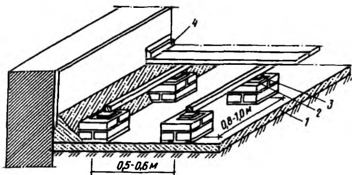
Рис. 8.7. Дощатый пол по кирпичным столбикам 1 — бетонная подготовка; 2 — два слоя рубероида или толя; 3 — осмоленная подкладка; 4 — плинтус
