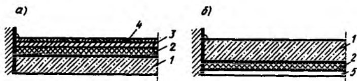
Рис. 8.40. Утепление перекрытия плитами из пенопласта 1 — плита перекрытия; 2 — плиты из пенопласта; 3 — цементная стяжка; 4 — покрытие пола; 5 — штукатурка
