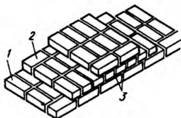
Рис. 5.8. Двурядная система кладки
