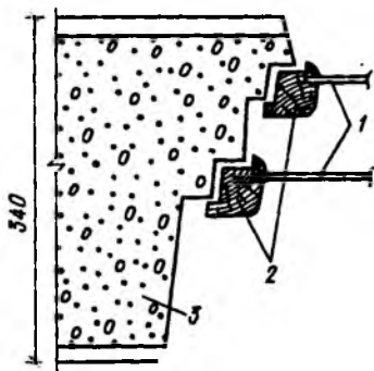
Рис. 6.4. Конструкция бескоробочного окна 1 — остекление; 2 — переплет; 3 — стена
