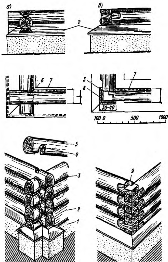
Рис. 5.1. Конструкции угловых врубок бревенчатых домов
