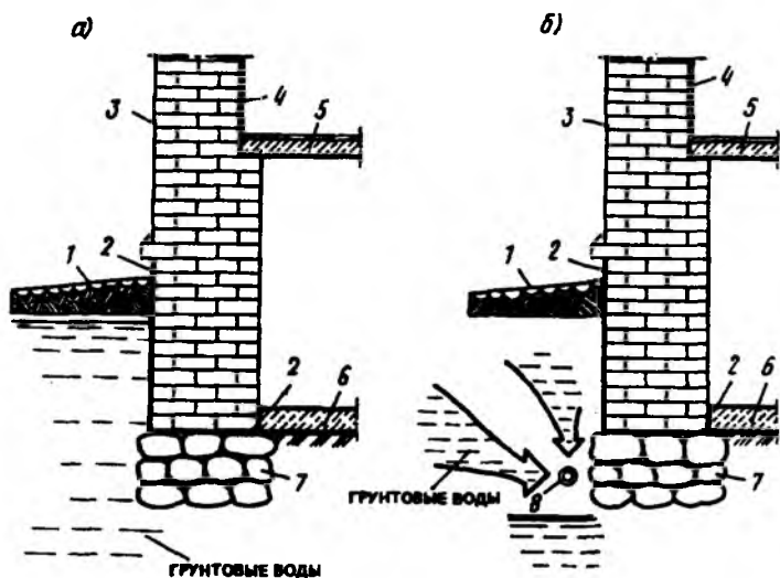
Рис. 2.22. Конструктивные мероприятия по защите от увлажнения грунтовыми водами стены подвального помещения
