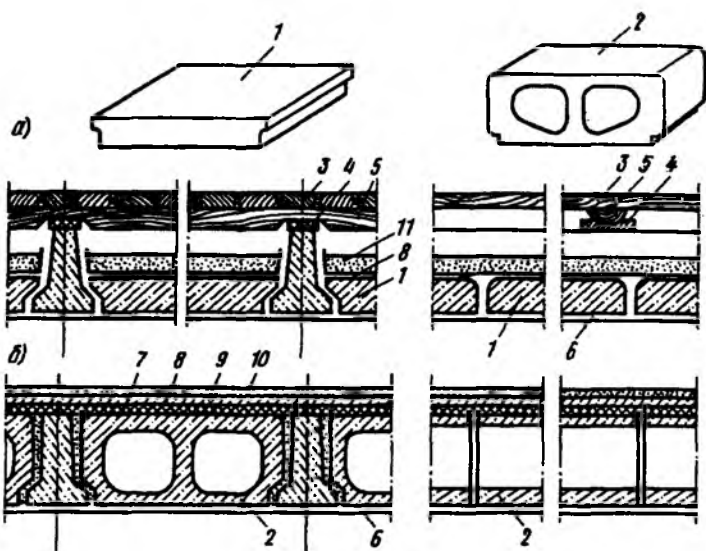
Рис. 8.26. Перекрытия по сборным железобетонным балкам с накатом из сплошных плит (а) и с заполнением двухпустотными вкладышами (б) 1 — гипсобетонная плита; 2 — легкобетонный вкладыш; 3 — дощатый пол; 4 — звукоизоляционная прокладка; 5 — лага; 6 — затирка; 7 — оргалит; 8 — толь; 9 — легкий бетон; 10 — чистый пол; 11 — засыпка (из шлака)
