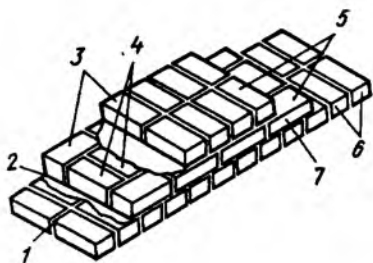
Рис. 5.7. Элементы кирпичной кладки
