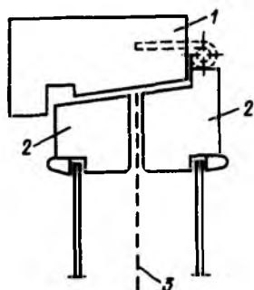
Рис. 6.27. Установка металлизированной пленки в межстекольном пространстве
