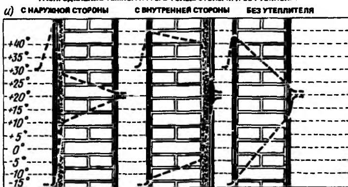
Рис. 5.22. Принципиальные схемы утепления наружных стен и распределение температуры в стене при утеплении их снаружи и изнутри 1 — слой пароизоляции; 2 — теплоизоляционный слой
