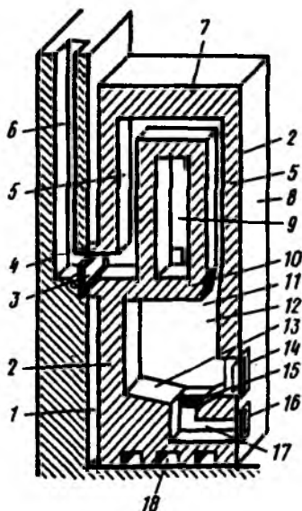
Рис. 9.1. Отопительная печь 1 — отступка; 2 — тепловоспринимающая поверхность; 3 — задвижка; 4 — патрубок; 5 — дымообороты; 6 — дымоход; 7 — перекрышка; 8 — теплоотдающая поверхность; 9 — тепловоздушная камера; 10 — свод печи; 11 — хайло; 12 — топочное пространство; 13 — под; 14 — топочная дверца; 15 — колосниковая решетка; 16 — поддувальная дверца; 17 — поддувало; 18 — шанцы
