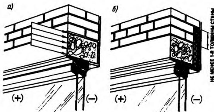
Рис. 5.36. Утепление стены над окном в зоне перемычки
