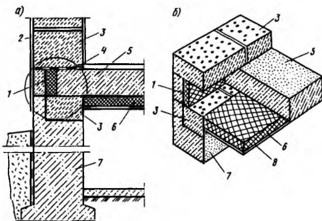
Рис. 8.43. Утепление цокольного перекрытия над подвалом a — разрез; б — фрагмент узла; 1 — утепление пенопластом; 2 — наружный отделочный слой; 3 — стеновой блок из керамзитобетона; 4 — гидроизоляция (цементный раствор); 5 — железобетонное перекрытие; 6 — плитный утеплитель (пенопласт); 7 — бетонная стена подвала; 8 — штукатурка
