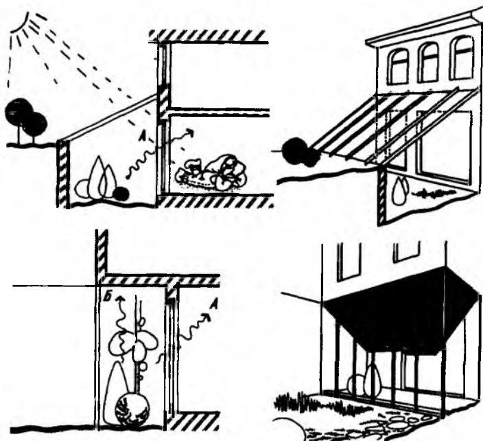
Рис. 10.7. Оранжерея около окон и стен цокольного этажа A — поток тепла в комнату через окно; B — поток тепла на второй этаж или через стык панелей с перекрытием
