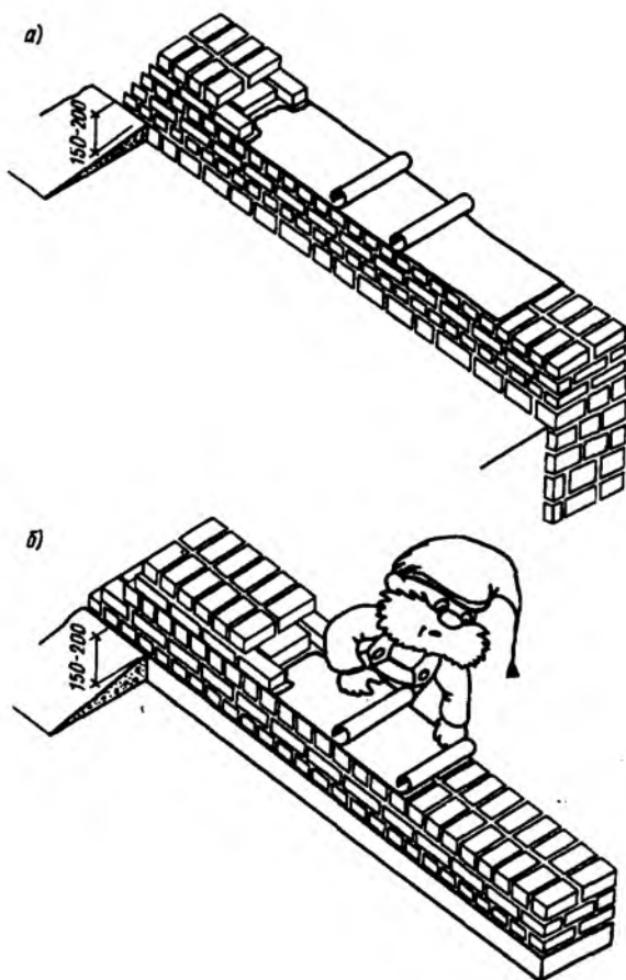
Рис. 8.20. Устройство гидроизоляции из двух слоев рубероида на битумной мастике (а) и двух слоев толя, уложенного насухо (б)
