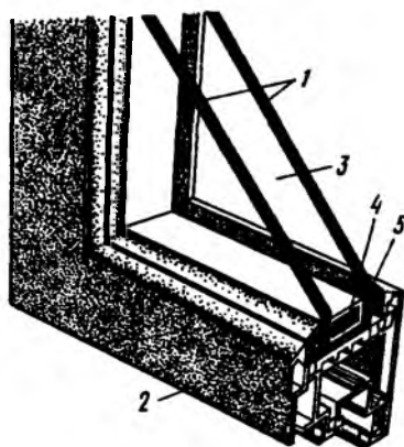
Рис. 6.3. Использование стеклопакета для остекления 1 — остекление; 2 — переплет; 3 — герметичная воздушная прослойка; 4 — распорный профиль; 5 — материал, впитывающий влагу из воздуха прослойки
