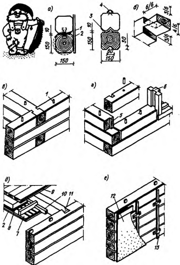
Рис. 5.4. Конструкция стены брусчатого дома
