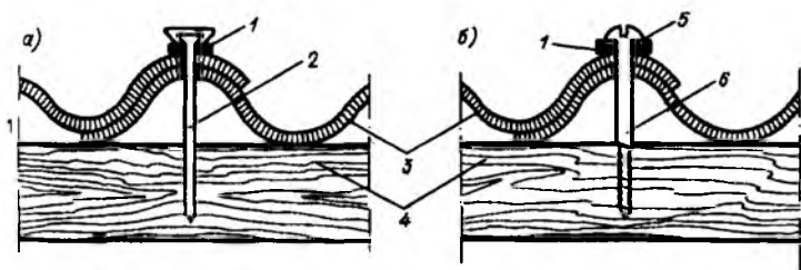
Рис. 7.17. Крепление волнистых асбестоцементных листов к обрешетке a — гвоздями (4—5)х(80—100) мм со шляпкой, покрытой оцинкованной сталью; b — шурупами (6—8)х(80—100) мм; 1 — мягкая прокладка; 2 — гвоздь; 3 — волнистый асбестоцементный лист; 4 — обрешетка; 5 — шайба; 6 — шуруп
