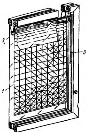
Рис. 6.28. Свертывающаяся штора 1 — экран; 2 — барабан; 3 — шнур
