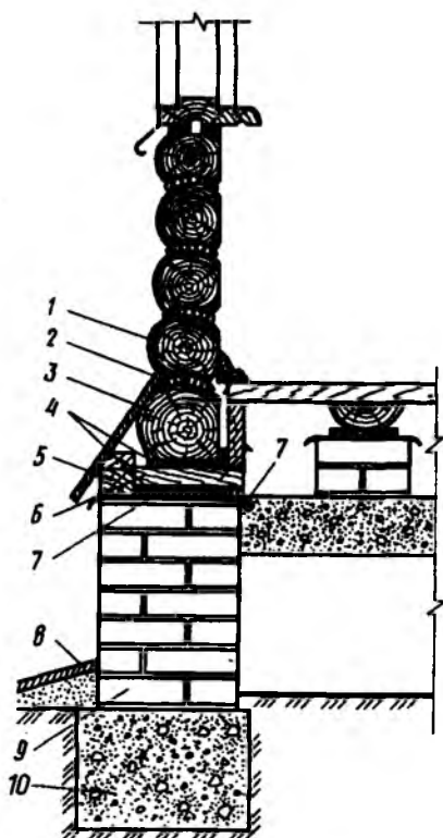
Рис. 5.3. Узел примыкания нижней обвязки рубленной стены к цоколю
