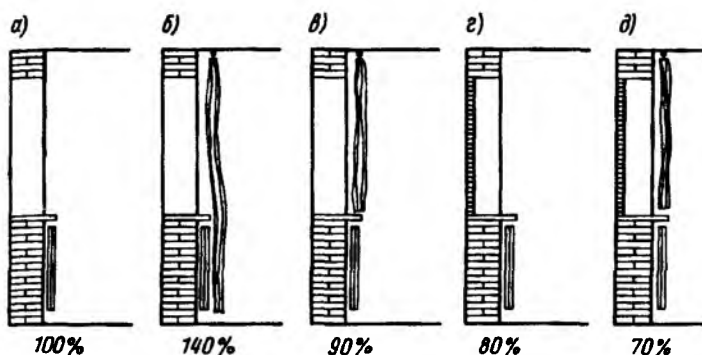
Рис. 6.24. Влияние зашторивания и экранирования окон на теплопотери, % а — окно без занавесок; б — окно с длинными занавесками, закрывающими отопительный прибор; в — окно с короткими занавесками, не закрывающими отопительные прибор; з — окно с экраном с наружной стороны остекления; д — окно с короткими занавесками и наружным экраном
