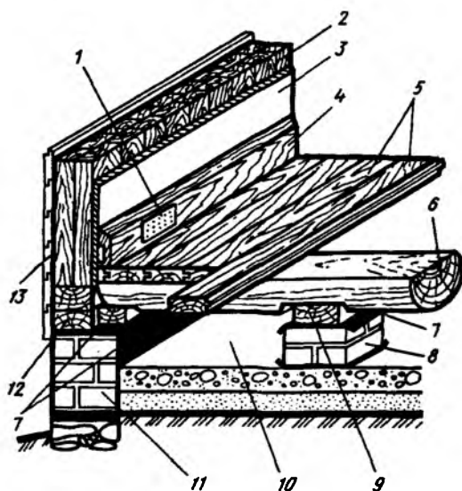
Рис. 8.12. Цокольные перекрытия при кирпичном цоколе и деревянных наружных стенах из досок
