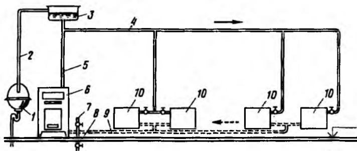
Рис. 9.10. Водяное отопление с прокладкой горячей линии под потолком, а обратной — у пола
