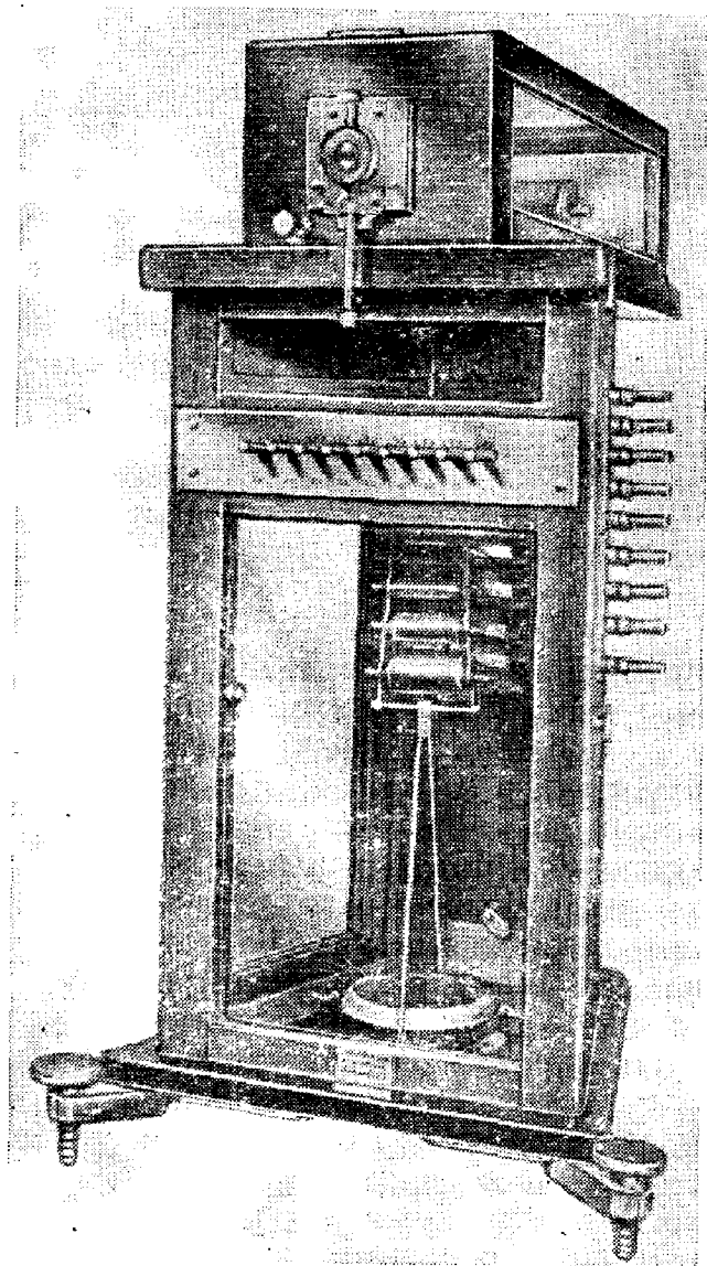
Весы конструкции Д. И. Менделеева (модель). ВНИИМ
