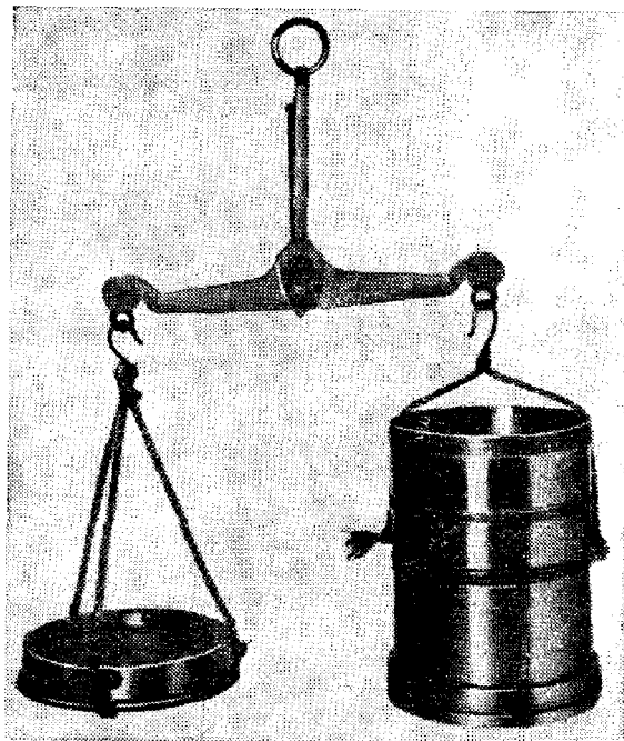
Пурка образцовая 5 фунтов 1889 г. ВНИИМ
