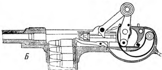
Р и с. 17. Пистолет сист. Борхардта: A — общий вид; B — схема подающего и запирающего механизмов.
