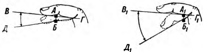
Р и с. 78. Преимущество спуска курка первой фалангой: движение пальца получается меньше.
