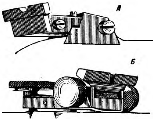
Рис. 43. Прицельные приспособления (прицелы) целевых спортивных пистолетов:
