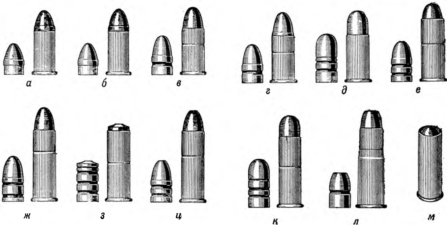
Рис. 47г. Образцы патронов в натуральную величину. Патроны центрального огня для револьверов: а — Кольта (короткий патрон), кал. 9 мм (38-го калибра); б — различных английских (Веблей, Бушльдог и др.), кал. 9 мм (38-го калибра); в — Кольта полицейского образца, кал. 9 мм (38-го калибра); г — Смит-Вессона, последнего полицейского образца, кал. 9 мм (38-го калибра); д — Смит-Вессона „специальный“ (усиленный патрон), средних дистанций, кал. 9 мм (38-го калибра); е — Кольта (длинный патрон), кал. 9 мм (38-го калибра); ж — Смит-Вессона „специальный“ (усиленный патрон), кал. 9 мм (38-го калибра); з — Смит-Вессона „специальный для дальних дистанций“ (усиленный патрон), кал. 9 мм (38-го калибра); и — Кольта, „специальный“ (последний образец), кал. 9 мм (38-го калибра); к — Кольта, „специальный полицейский“ (последний образец), патрон, так называемый „38-40“, кал. 9 мм (8-го калибра); л — Винчестера (известный охотничий патрон, так называемый „38-40“), кал. 9 мм (8-го калибра); м — Смит-Вессона для целевых револьверов и пистолетов (короткобойный патрон), кал. 9 мм (38-го калибра).
