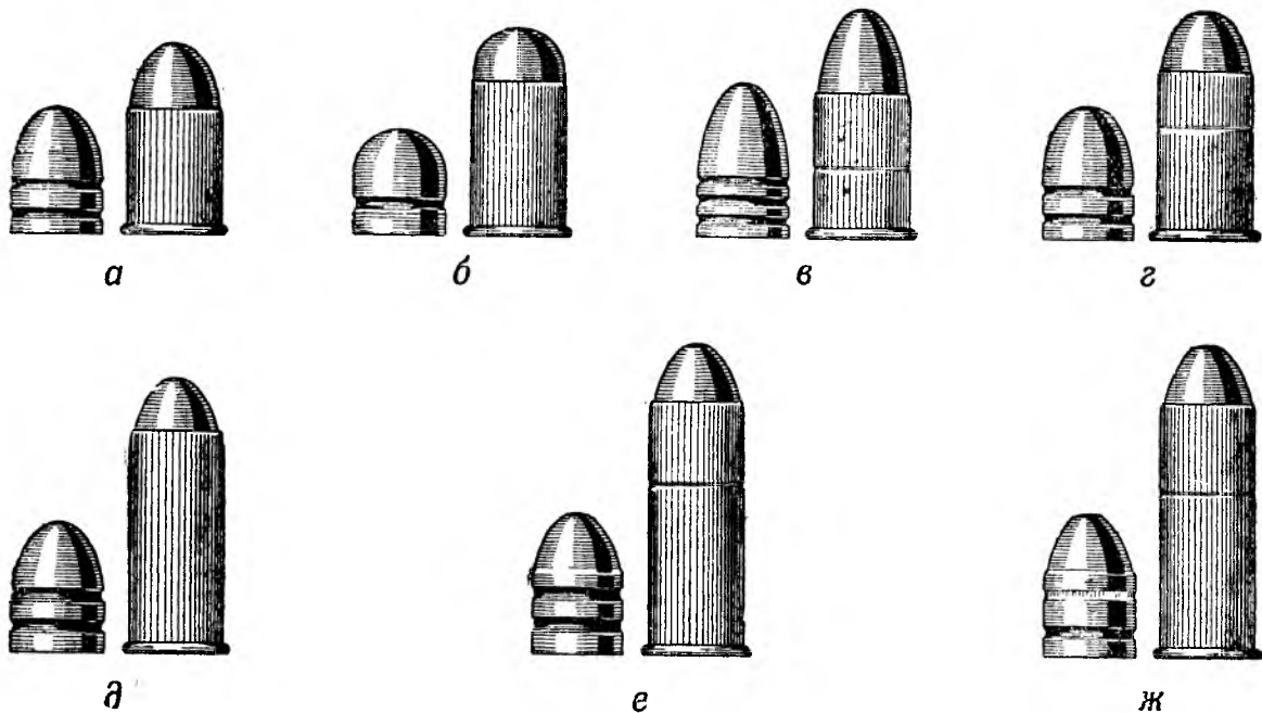
Р и с. 47е. Образцы патронов в натуральную величину. Патроны центрального огня для револьверов: а — различных английских (Булльдог, Скотт и др.), кал. 11,43 мм (450-го калибра); б — Веблей, кал. 11,43 мм (450-го калибра); в — Веблей, армейская модель (II образца), кал. 11,5 мм (450-го калибра); г — автоматических (45 230) английских, кал. 11,5 мм (455-го калибра); д — Смит-Вессона, кал. 11,43 мм (5-го калибра); е — Кольта, кал. 11,43 мм (45-го калибра); ж — казенного образца 1909 г. (США), кал. 11,43 мм (45-го калибра).
