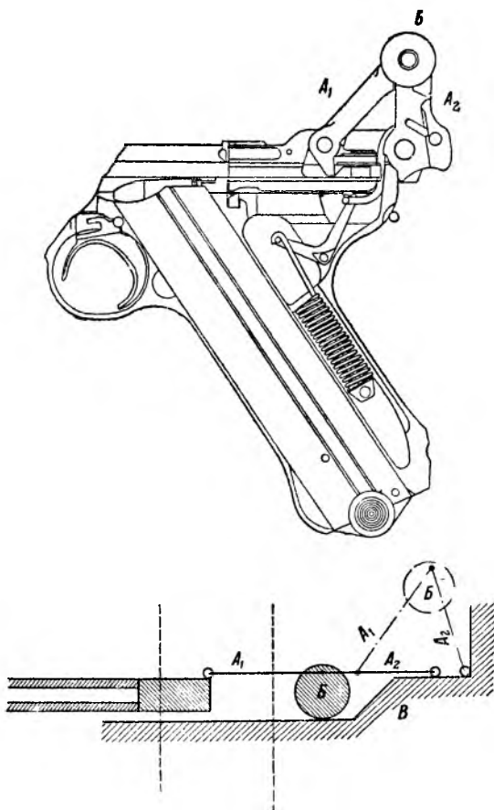
Рис. 20. Схема запирающего механизма пистолета „Парабеллюм“.
