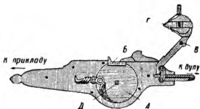
Р и с. 7. Немецкий колесцовый замок первой половины XVI в.
