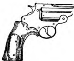
Р и с. 91. Крючок на спусковой скобе для задержки среднего пальца правой руки.
