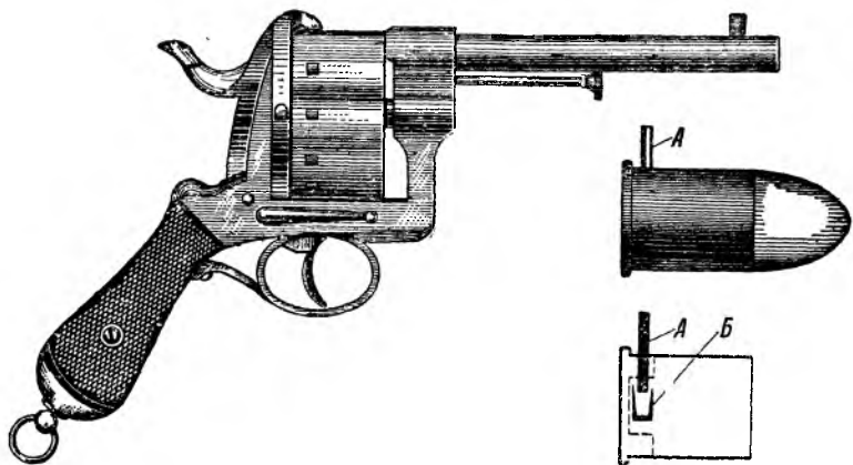
Рис. 15. Револьвер, патрон и гильза (в разрезе) сист. Лефшоэ обр. 1846 г.:
