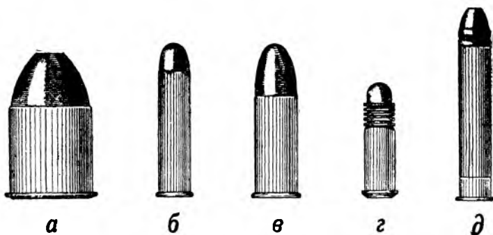
Р и с. 47 ж. Образцы патронов в натуральную величину. Различные патроны, под которые строятся револьверы и пистолеты: а — Элей (для двухствольных охотничьих „медвежьих“ пистолетов), кал. 15 мм (577-го калибра), б — Велодог, кал. 5,75 мм (22-го калибра); в — швейцарский казенный образец, кал. 7,7 мм (30-го калибра); г — „Long Rifle 22“ (известный малокалиберный патрон бокового огня), кал. 5,6 мм (22-го калибра); д — так называемый „франсеф“, длинный малокалиберный патрон бокового огня (французский), применяется для револьверов (Велодог, Франкотт и др.) и целевых пистолетов кал. 6 мм.
