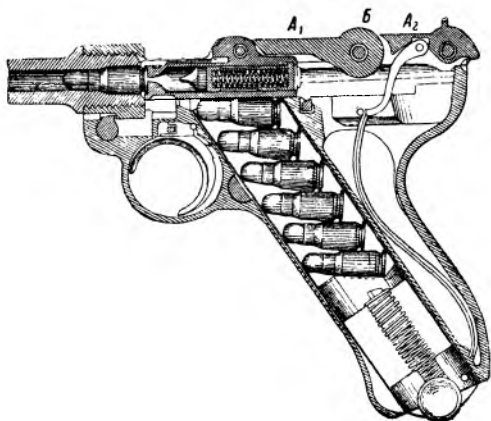
Р и с. 19. Продольный вертикальный разрез пистолета „Парабеллум“ обр. 1900 г.
