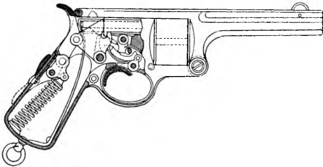
Р и с. 38. Автоматический револьвер военного образца сист. Коломбо-Риччи (Италия) в разрезе.
