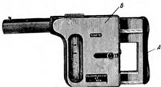
Рис. 41а. Оригинальный неавтоматический пятизарядный pistol сист. Галлюа. Чтобы произвести из него выстрел, нужно, захватив pistol кистью руки, вжимать подвижную раму (А) в корпус pistol та (В).
