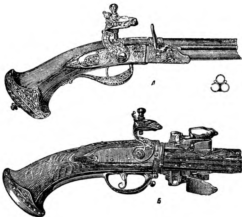
Рис. 10. Трехствольный (А) и двухствольный (Б) ударно-кремневые пистолеты-револьверы; последний показан в момент поворота стволов на 90^\circ , поэтому видны обе полки.
