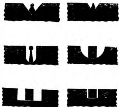
Рис. 70. Прицельные приспособления револьверов и пистолетов (основные типы).
