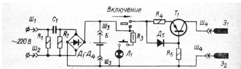
Рис. 54. Электрическая схема ионизатора ЛК-26а:
