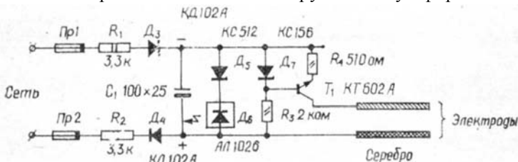
Рис. 59. Электрическая схема ионатора ЛК-29.
