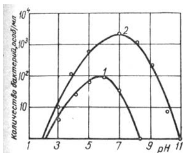
Рис. 9. Влияние pH на обеззараживающий эффект серебра:
