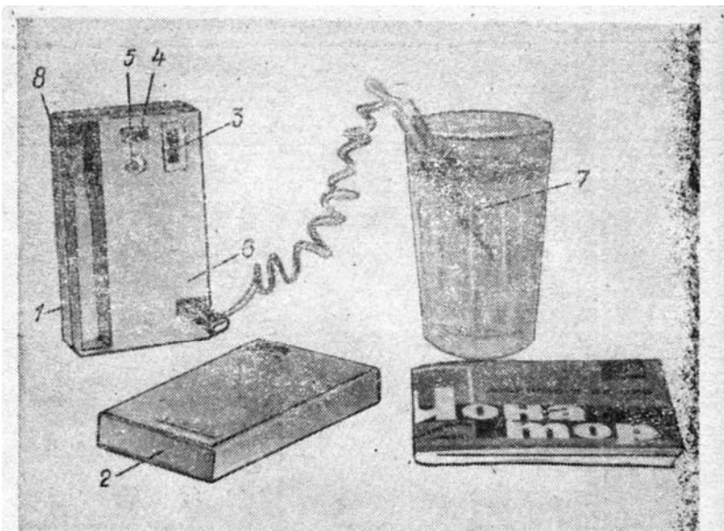
Рис. 53. Ионизатор ЛК-26а («Турист-2») — модель, выпускаемая Сумским заводом электронных микроскопов:
