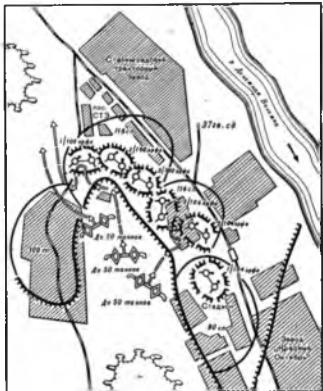
Схема 7. Боевые действия 100-й и 104-й отдельных рот фугасных огнеметов в оборонительных боях за Сталинград в октябре 1942 г.
