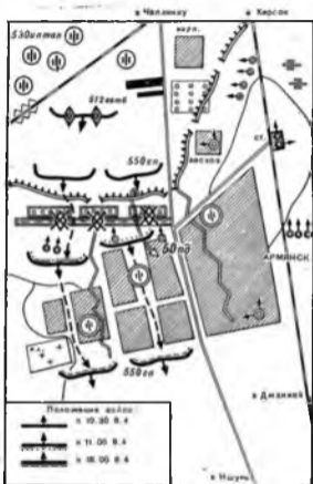
Рис. 44. Боевые действия 512-го отдельного инженерно-танкового батальона при прорыве обороны противника и освобождении Армянска
