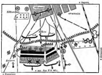
Схема 45. Боевые действия 512-го отдельного огнеметно-танкового батальона в ночной атаке при освобождении Джульги в апреле 1944 г.
