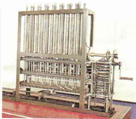
Вычислительная машина, созданная в Англии в 1922 г., являлась шестицифровым калькулятором, способным производить вычисления и печатать цифровые таблицы
