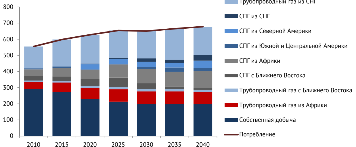
Рисунок 2.32. – Баланс газа на рынке Европы
