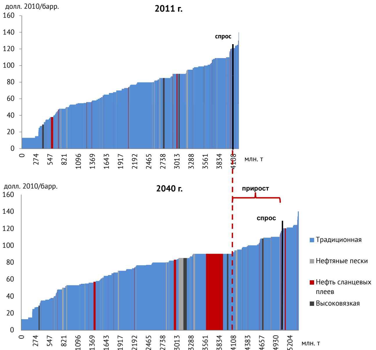
Рисунок 2.11. – Кривая предложения (цена производства) нефти
