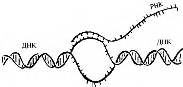
Перевод информации с ДНК на однополосный «передатчик» РНК (по Кэлледайну, 2004, с. 65)
