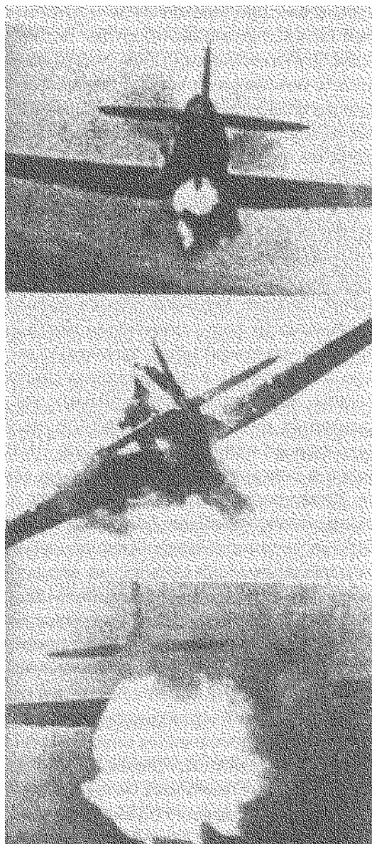
Один из немногих примеров удачной работы фотопулемета: несколько кадров сбития немецкого истребителя «Me.109G», 1944 г.
