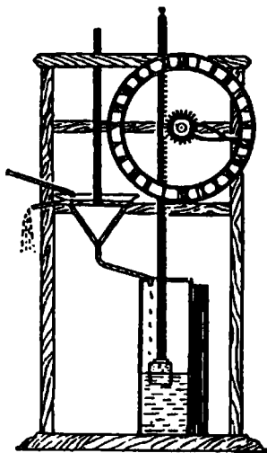
Клепсидра. Устройство клепсидры
