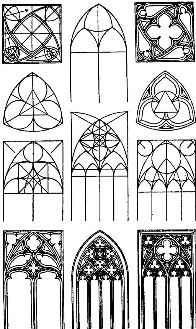
Арка. Геометрия готических арок
