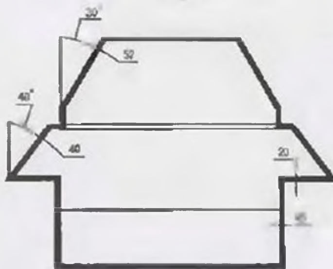
Средний танк Т-34. Схема бронирования
